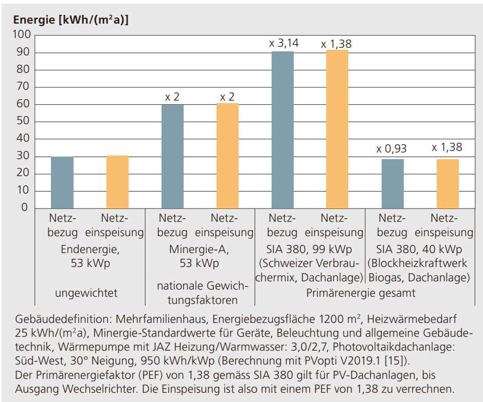
Abbildung 1.22: Benötigte Photovoltaikleistung, um die Null-Energiebilanz mit unterschiedlichen Gewichtungsfaktoren zu erreichen. Umrechnungsfaktoren für Strom gemäss den nationalen Gewichtungsfaktoren [13] und Norm SIA 380 [14].
