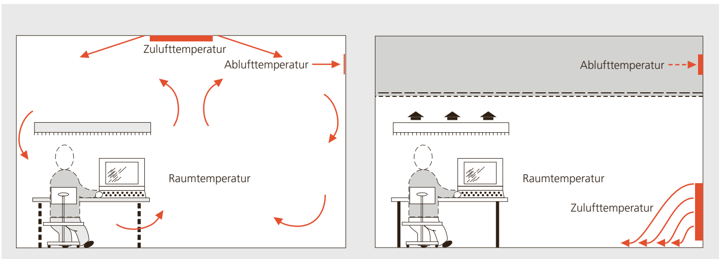
Abbildung 4.15: Mischlüftung (links) und Quelllüftung (rechts). (Quelle: Lindab)
