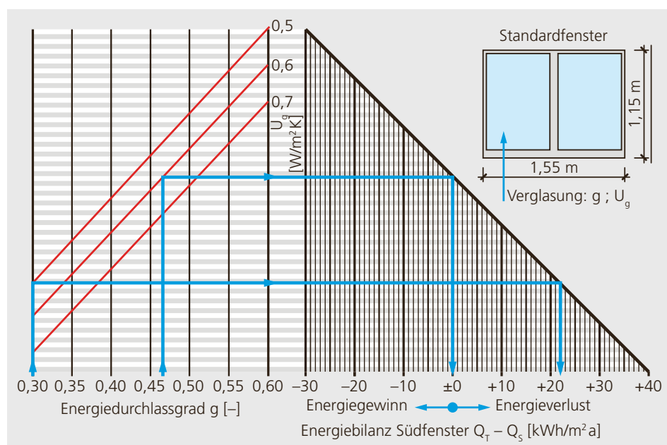
Abbildung 3.24: Energiebilanz bei Südfenster, also Transmissionswärmeverlust minus Energiegewinn durch Sonneneinstrahlung, in Abhängigkeit vom Energiedurchlassgrad g und vom Glas-U-Wert U_g . Sonnenschutzgläser mit g -Wert 0,3 führen selbst bei Dreifach-IV mit U_g = 0,5 W/(m^2 K) zu einem bilanzierten Energieverlust. Ab einem g -Wert von 0,47 führen Dreifach-IV mit U_g = 0,6 W/(m^2 K) zu einem bilanzierten Energiegewinn.
