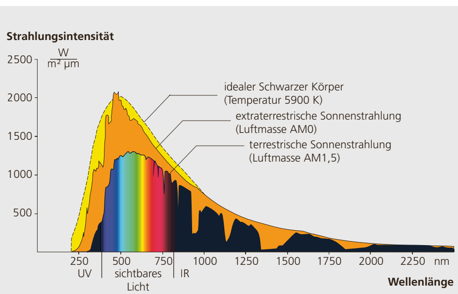
Abbildung 2.21: Solarspektrum mit Wellenlängenbe- reich des sichtbaren Lichtes. (Quelle: Wikimedia)
