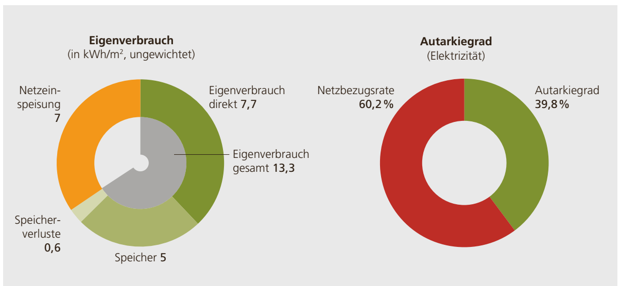
Abbildung 4.41: Eigenverbrauch und Autarkiegrad für ein Einfamilienhaus im schweizerischen Mittelland mit 200m 2 Energiebezugsfläche, einer optimal ausgerichteten PV-Anlage von 25 m 2 mit Batteriespeicher von 5 kWh Kapazität. (Quelle: Gerechnet mit Minergie-Rechentool PVopti)
