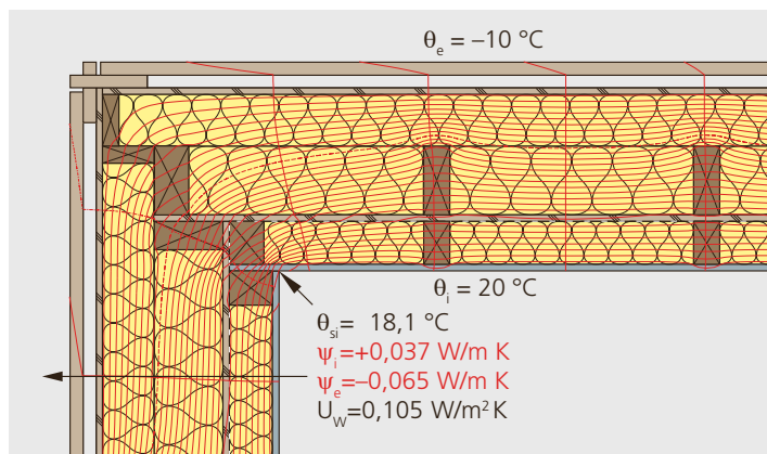
Abbildung 3.25: Beim Zusammenbau von Holzbauteilen führen die geometrie- und materialbedingten Einflüsse zu keinen erhöhten Wärmeflüssen (bezogen auf die Aussenabmessung).
