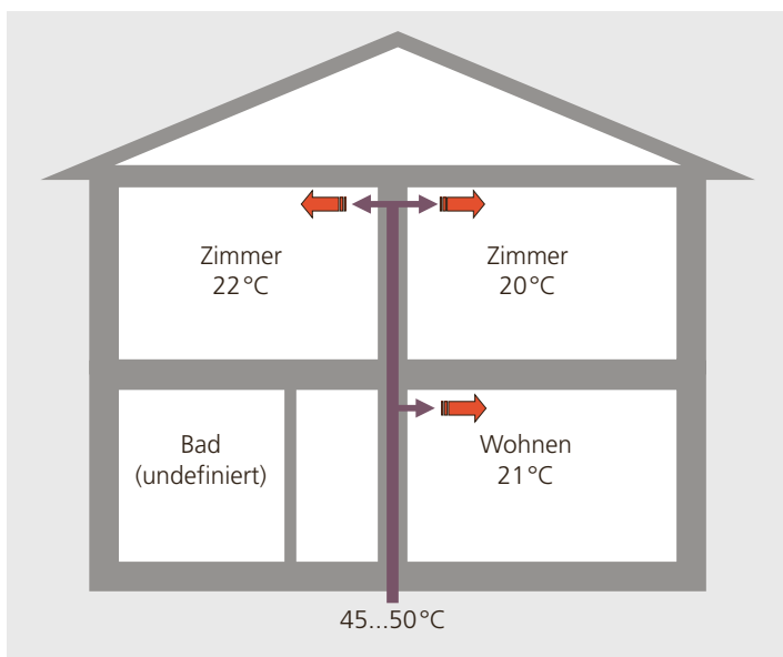
Abbildung 4.3: Prinzip Heizung mit Zuluft.
