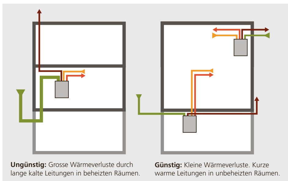
Abbildung 4.17: Skizze mit günstiger und ungünstiger Anordnung.
