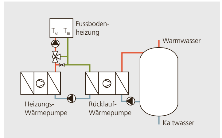
Abbildung 4.6: Schema RL-Wärmepumpe.
