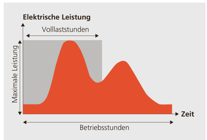
Abbildung 4.31: Volllaststunden nach SIA 387/4.
