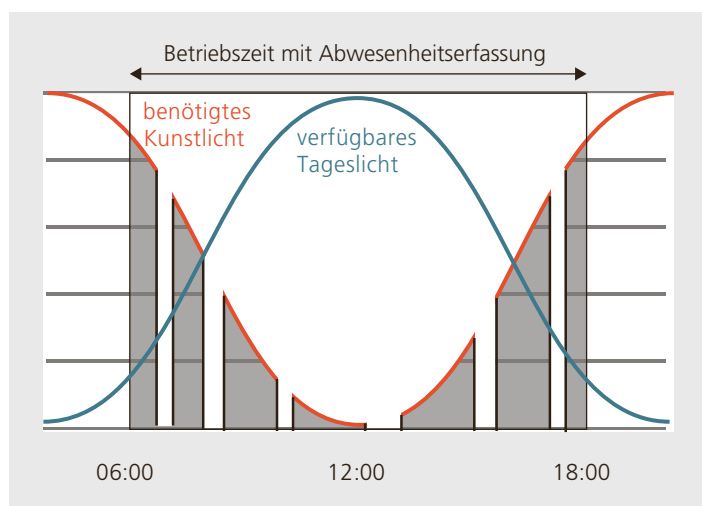
Abbildung 4.33: Durch geeignetes Lichtmanagement kann viel Energie eingespart werden. (Quelle: Trilux)
