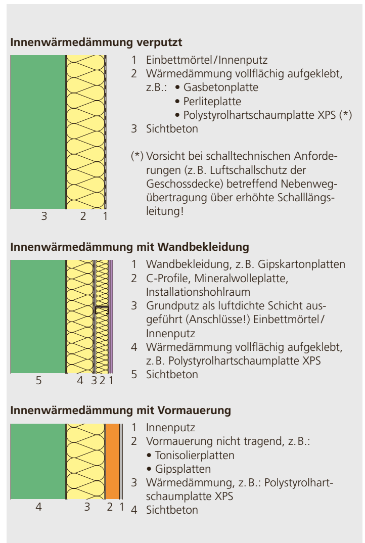
Abbildung 3.16: Konstruktionsbeispiele für innen wärmedämmte Sichtbeton-Aussenwände.
