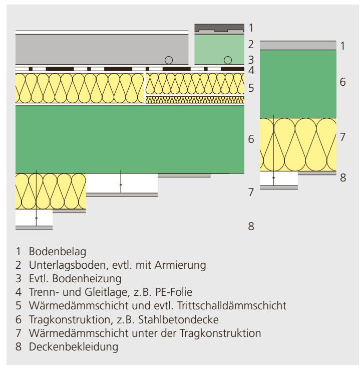
Abbildung 3.20: Bo- denkonstruktion über Aussenluft und nicht beheizten Räumen mit unter- schiedlicher Anord- nung der Wärme- dämmschicht und Massnahmen, um den Trittschall- schutz zu gewähr- leisten.
