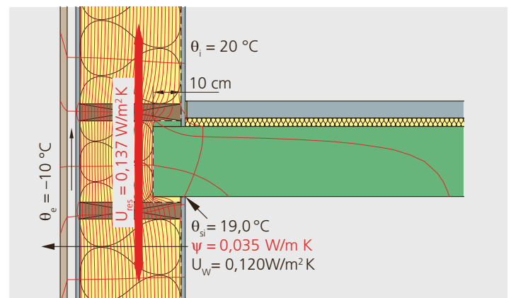
Abbildung 3.26: Beim Hybridbau sind Wärmebrückenverluste über die in das Aussenwandelement hineinragenden Geschossdecken und Trennwände aus Stahlbeton unvermeidbar. Der Wärmebrückeneinfluss des energetisch und schalltechnisch optimierten Details hält sich aber in Grenzen.
