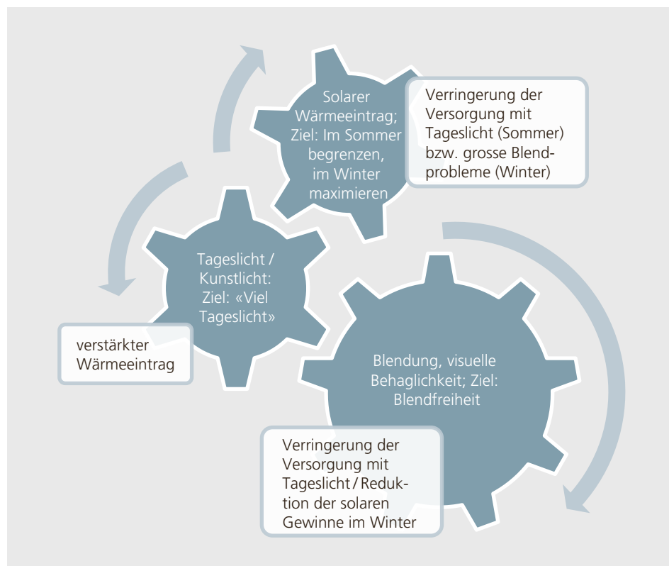
Abbildung 2.30: Spannungsdreieck zwischen den Zielen optimale Tageslicht- versorgung, Blend- freiheit und Wär- meeinträge – die Wärmeeinträge sind zudem im Win- ter zu maximieren und im Sommer zu minimieren.
