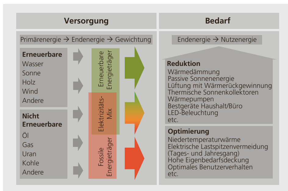
Abbildung 1.7: Bedarfs- und Versorgungsseite von Energie in Gebäuden. Schematische Darstellung der direkten Optimierungsfelder des Gebäudes und der erforderlichen Energiezufuhr von aussen des Gebäudes.
