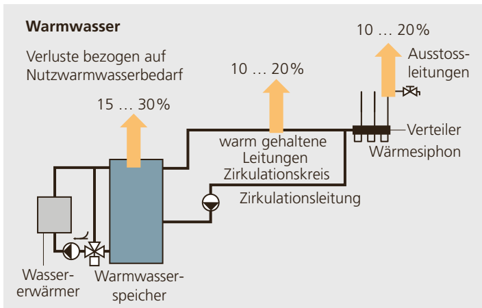
Abbildung 4.5: Verluste bei Warmwasseranlagen.
