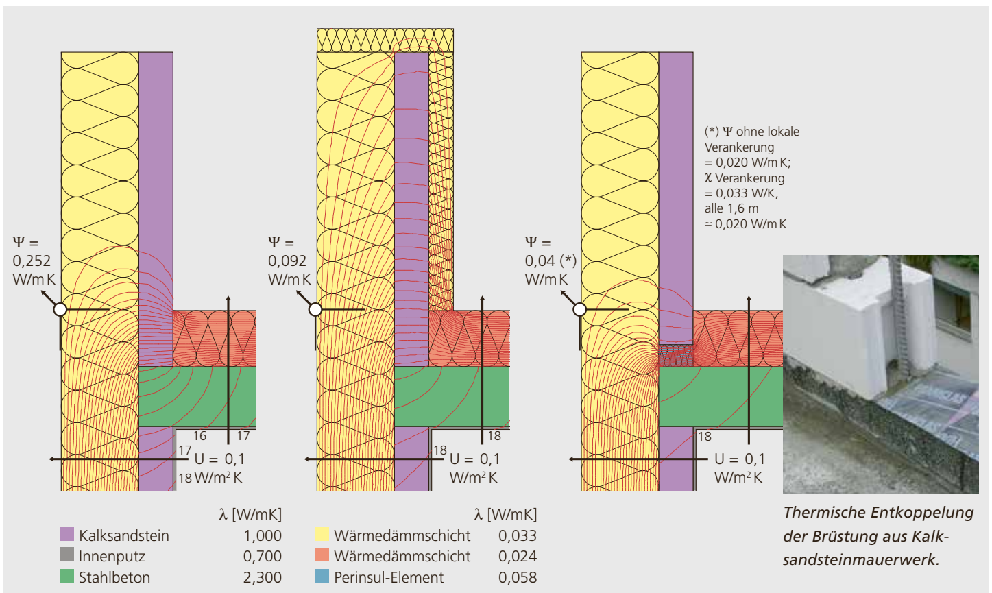
Abbildung 3.31: Selbst eine überdämmte Attikabrüstung verursacht noch eher hohe Wärmebrückenverluste. Optimal ist es, die Brüstung auf ein Wärmedämmelement zu stellen und dadurch thermisch von der Stahlbetondecke zu entkoppeln.
