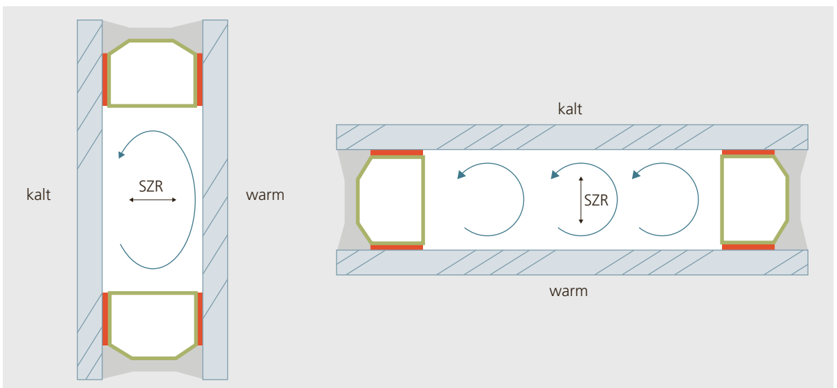
Abbildung 2.18: Erhöhter konvektiver Wärmetransport bei geneigten Gläsern – sogenannte Rayleigh-Bénard-Konvektion. (Quelle: ift Rosenheim)
