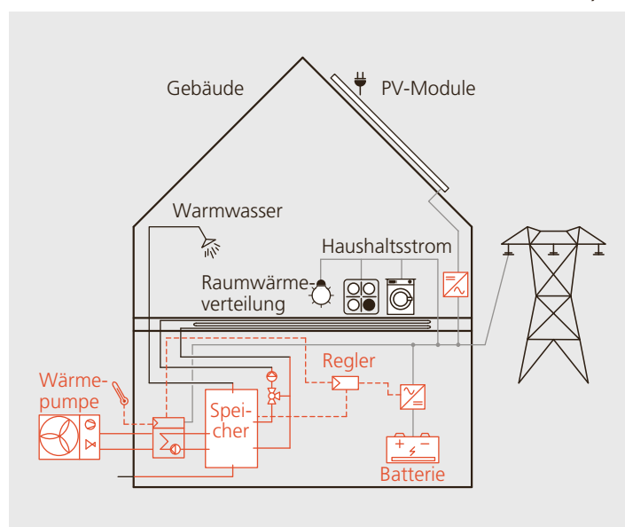
Abbildung 4.42: Ein Wohngebäude mit allen Komponenten zur Energieversorgung mit einem hohen Eigenverbrauchsanteil (Regler, Speicher, Batterie, Wärmepumpe, PV-Anlage und Netzanschluss). (Quelle: SPF Institut für Solartechnik)
