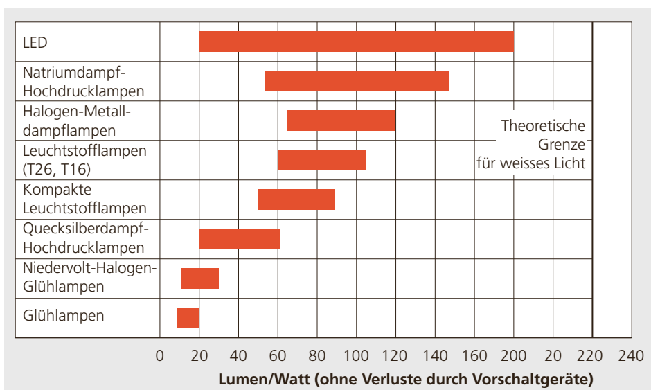
Abbildung 4.28: Lichtausbeuten von unterschiedlichen Leuchtmitteln. (Quelle: Licht.de)
