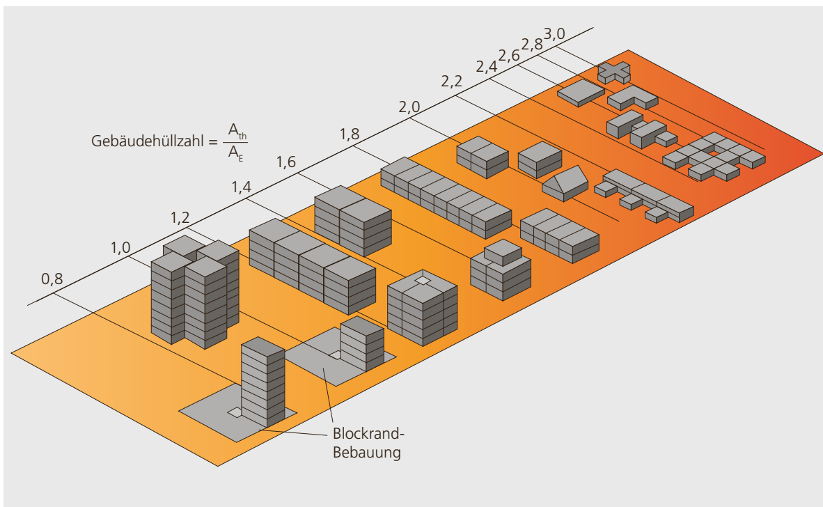
Abbildung 2.1: Kompaktheit und Gebäudehüllzahl. (Quelle: Solarfibel, Wirtschaftsministerium Baden-Württemberg)
