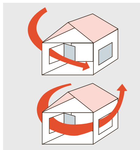
Abbildung 2.27: Einseitige Lüftung (oben) und Querlüftung (unten). (Quelle: Fenster Keller AG)
