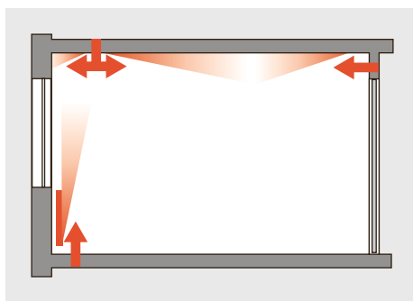
Abbildung 4.12: Lage von Zuluft- Durchlässen; der Zu- luftstrahl darf nicht in den Aufenthalts- bereich gerichtet sein.
