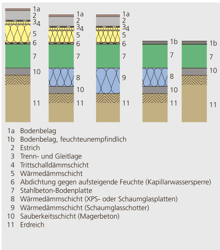
Abbildung 3.22: Bodenkonstruktion über Erdreich, mit unterschiedlicher Anordnung der Wärme-/Trittschalldämmschichten über und unter der Betonbodenplatte, je nach Anforderung an den Wärme- und Trittschallschutz.
