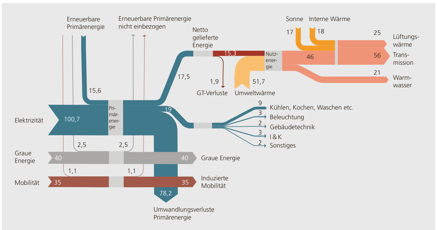
Abbildung 1.14: Spezifische Energieflüsse in kWh pro m 2 EBF pro Jahr in einem durchschnittlichen Mehrfamilienhaus-Neubau mit einer Erdsonden-Wärmepumpenanlage für Heizung und Warmwasser.
