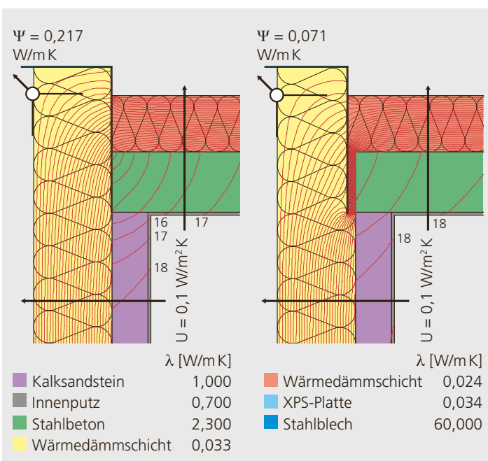
Abbildung 3.29: Durchgehende Tragbleche aus Stahlblech führen beim Dachrand zu hohen Wärmebrückenverlusten. Diese können durch eine thermische Trennung mit einer 3 \text{ cm} dicken druckfesten XPS-Platte um Faktor 3 reduziert werden.
