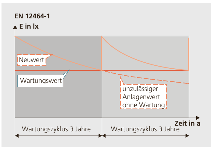
Abbildung 4.30: Verlauf der Beleuchtungsstärke einer Anlage über die Betriebszeit. (Quelle: Trilux)
