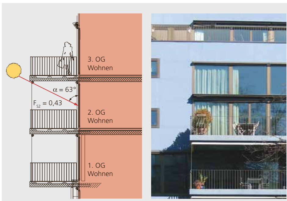
Abbildung 3.3: Durch die Balkone werden die gegen Süden orientierten Fenster erheblich verschattet. Über die Heizperiode betrachtet führt die Fensterfront hinter den Balkonen zu einem bilanzierten Energieverlust von 33 \text{ kWh}/\text{m}^2 . Ohne verschattende Balkone resultiert ein Energiegewinn von 19 \text{ kWh}/\text{m}^2 . Die Differenz von 52 \text{ kWh}/\text{m}^2 Fensterfläche entspricht dem Heizwert von etwa 5 Litern Heizöl.
