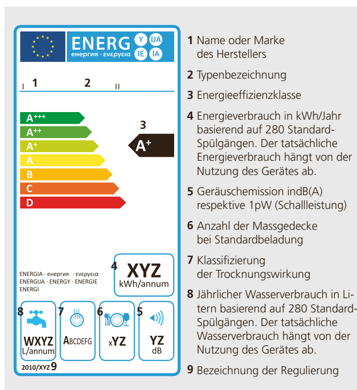
Abbildung 4.20: Energieetikette eines Geschirrspülers als Beispiel. (Quelle: Energie-Schweiz)
