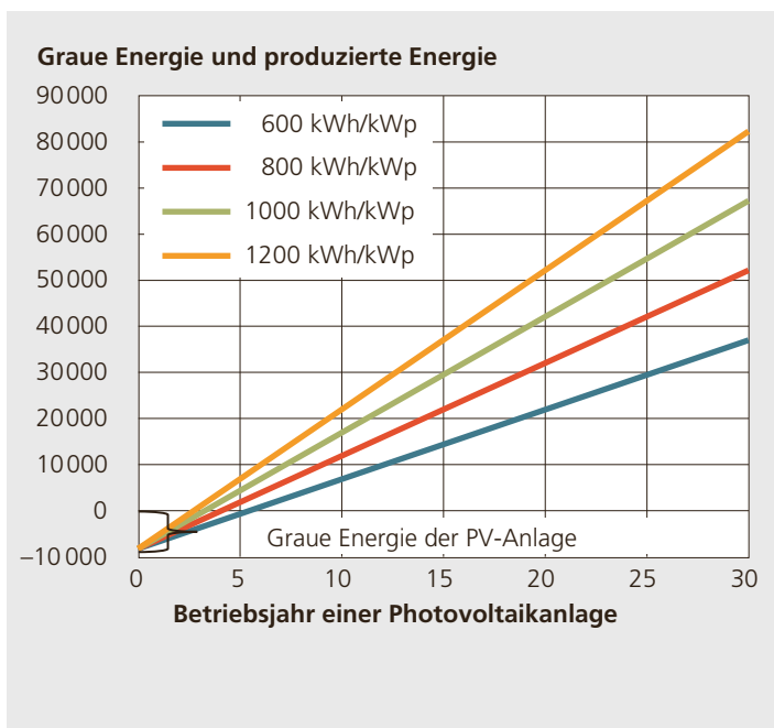
Abbildung 1.30: Amortisationszeit von Photovoltaikanlagen und eingesparte nicht erneuerbare Primärenergie durch den Ertrag (graue Energie: 7390 kWh/kWp, f_{nren,CH-Verb.Mix} = 2,52 , f_{nren,PV\text{Ertrag}} = 0,289 , basierend auf KBOB-Ökobilanzdatenbank 2016, Degradation 0,5% pro Jahr).
