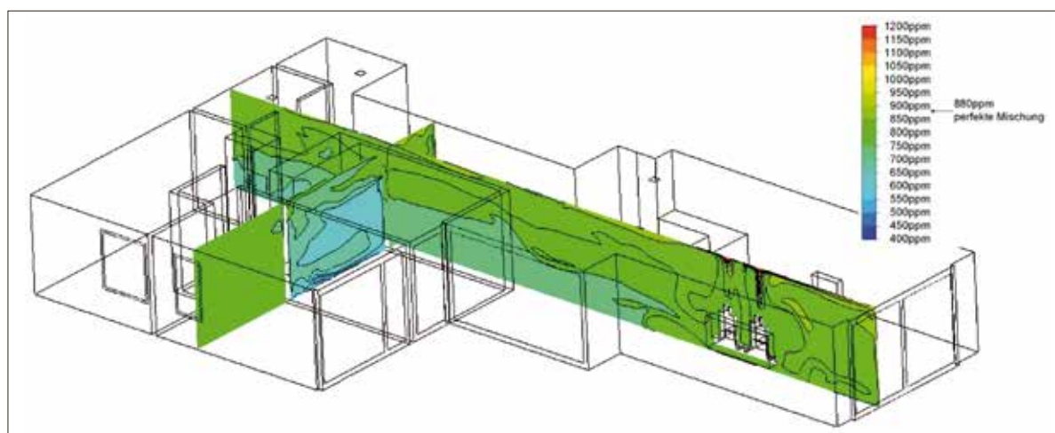
Abbildung 4.14: CO 2 -Konzentration bei freier Durchströmung des Wohnzimmers. (Quelle: AHB 09)
