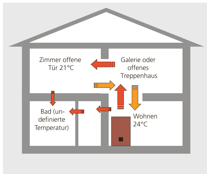
Abbildung 4.4: Prinzip Ofen mit freier Wärmeverteilung.
