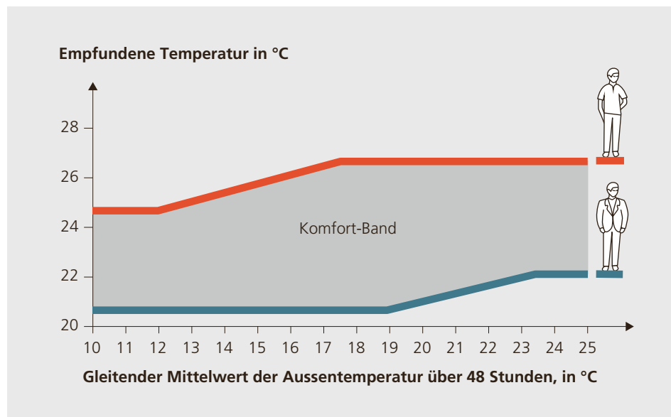
Abbildung 4.46: Norm SIA 382/1:2014 und Norm SIA 180:2014, Komfortbänder (Grafik: FHNW, J. Bichsel). Lesebeispiel: Bei einem gleitenden Mittelwert der Aussentemperatur über 48 Stunden von 23,5°C liegt das Temperatur-Komfortband zwischen 22°C (Bekleidung: Business-Anzug mit Krawatte) und 26,5°C (Bekleidung: lange Hose und Kurzarm-Hemd).
