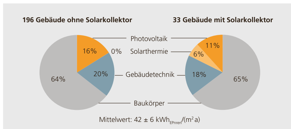
Abbildung 1.26: Anteil von Gewerken an der grauen Energie von 229 Minergie-A-Gebäude mit und ohne Solarthermie (Stand 2012).
