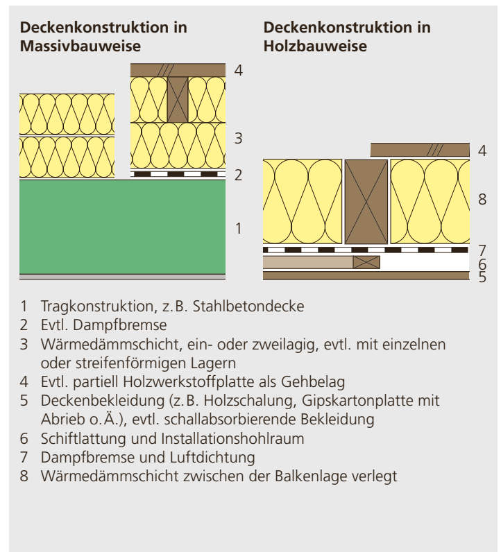
Abbildung 3.23: Deckenkonstruktion gegen unbeheizten Dach- oder Estrichraum, evtl. nicht oder nur beschränkt begehbar.
