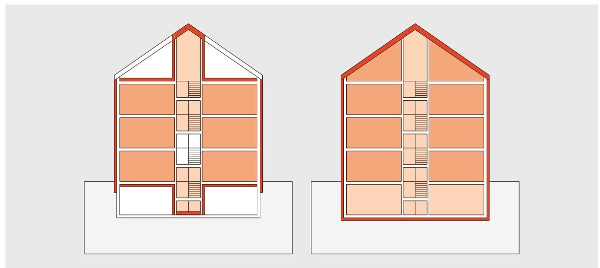
Abbildung 2.3: Verlauf der thermischen Gebäudehülle, links Keller und Dach ausserhalb der thermischen Hülle, rechts Keller und Dach in der thermischen Gebäudehülle.
