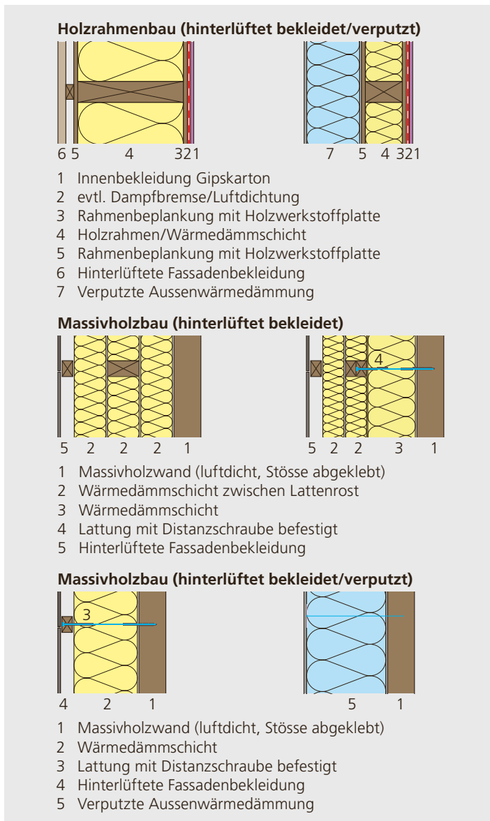
Abbildung 3.17: Konstruktionsbeispiele für Holzbau-Aussenwände.
