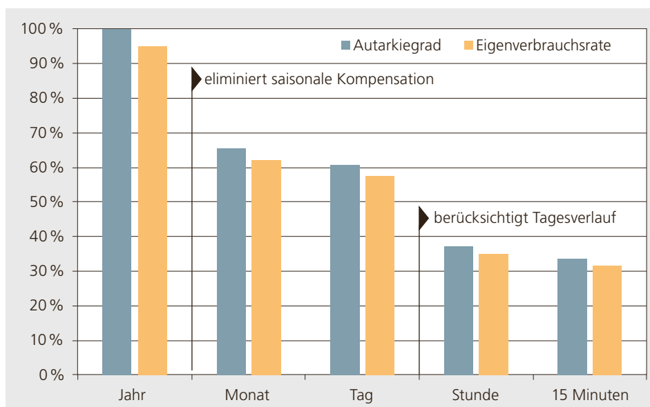
Abbildung 1.21: Autarkiegrad und Eigenverbrauchsrate in Abhängigkeit von der zeitlichen Auflösung, Basis 15-Minuten-Werte. Ertrag: 11 200 kWh/a, Verbrauch 10 600 kWh/a. (Quelle: [12])
