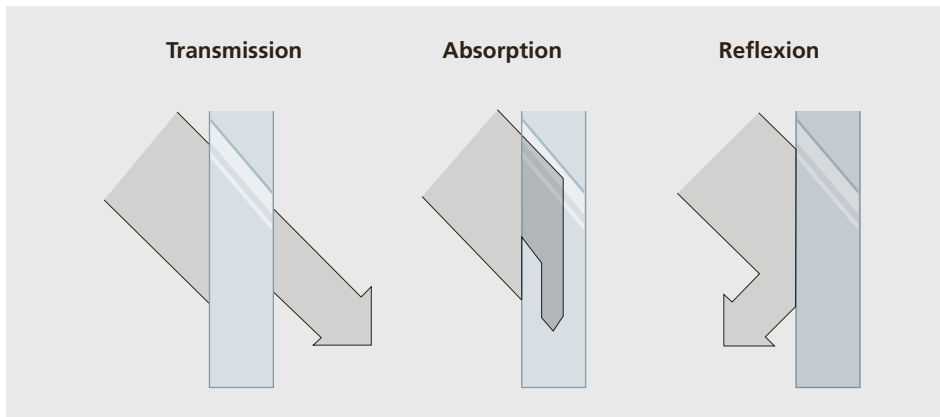
Abbildung 2.19: Vorgänge beim Auftreffen von kurzwelliger Strahlung auf ein Bauteil. (Quelle: Glas Trösch)
