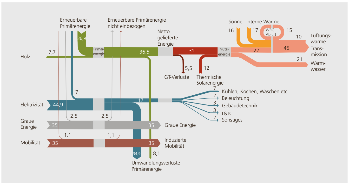
Abbildung 1.15: Spezifische Energieflüsse in kWh pro m 2 EBF pro Jahr im Mehrfamilienhaus-Neubau im Minergie-Standard.
