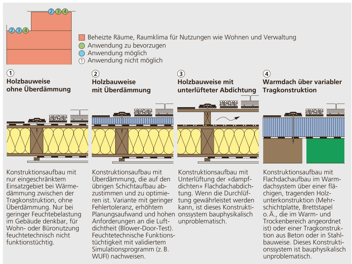
Abbildung 3.8: Konstruktionssystematik Flachdächer bei Holzbaukonstruktion und über Tragkonstruktion aus Beton/Stahlbau. Die feuchtetechnische Funktionstüchtigkeit der Holzbauvarianten 1 und 2 muss unter Berücksichtigung der dynamischen Effekte, z. B. mittels «WUFI», erfolgen; die Variante 1 ist jedoch nur bei geringer Feuchtebelastung möglich.
