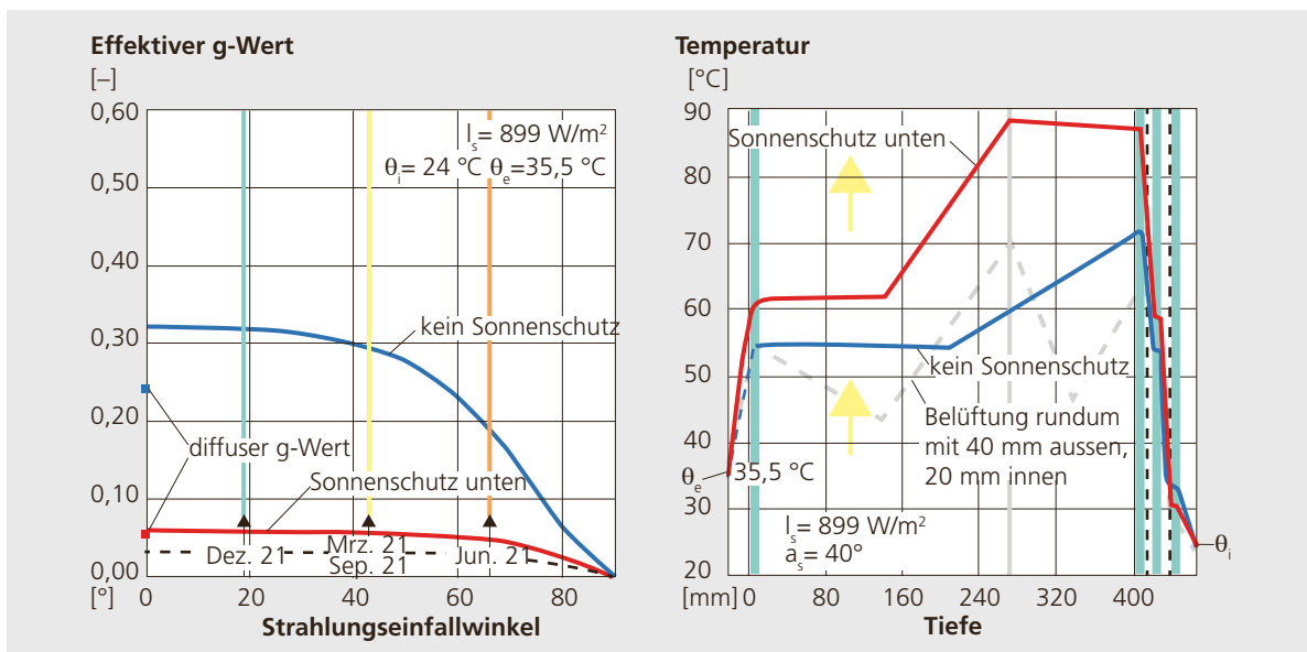
Abbildung 2.23: Effektiver g-Wert für direkte und diffuse Strahlung mit und ohne Lamellenstore in Abhängigkeit vom Profilwinkel (links) und Temperaturen in den Bauteilebenen für einen Sonnenhöhenwinkel von 40° (Maximalwerte, rechts).
