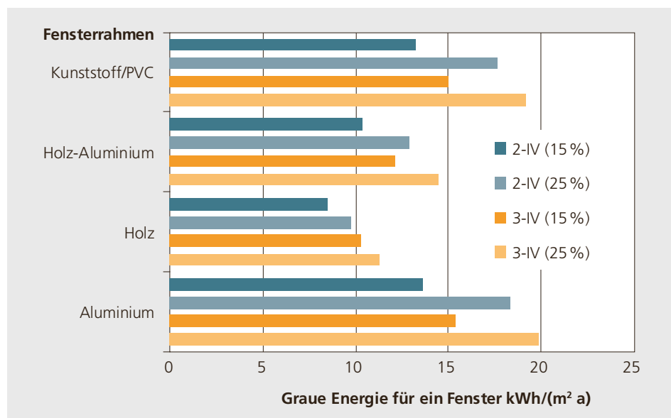
Abbildung 1.27: Graue Energie von zwei- und dreifach verglasten Fenster mit verschiedenen Rahmenmaterialien und -anteilen, Amortisationszeit 30 Jahre (KBOB-Ökobilanzdatenbank 2016, nicht erneuerbare Primärenergie, 2-IV: U_g = 1,1 \text{ W/(m}^2 \text{K)} , Dicke 18 mm, 3-IV: U_g = 0,6 \text{ W/(m}^2 \text{K)} , Dicke 40 mm).
