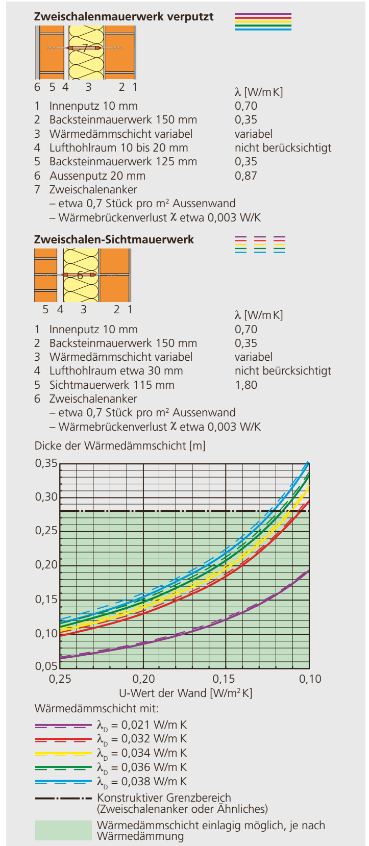
Abbildung 3.14: Zweischalenmauerwerk verputzt oder Sichtmauerwerk.
