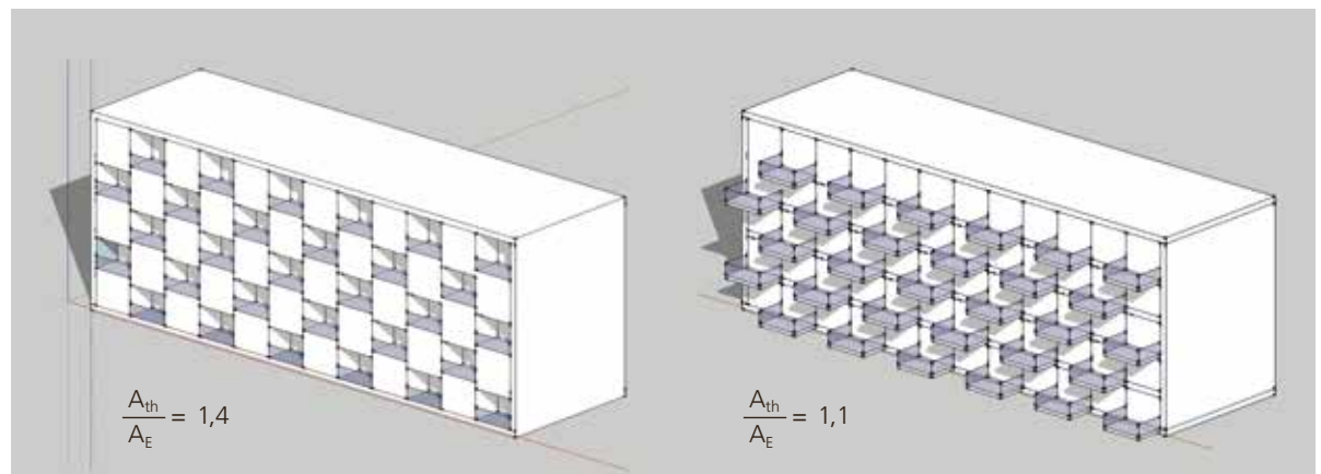
Abbildung 2.2: Das Gebäudevolumen mit den Loggien wirkt recht kompakt, hat aber auf der Südfassade 111 % mehr Gebäudehüllfläche. Bei gleicher Energiebezugsfläche hat das Gebäude mit Loggien eine Gebäudehüllzahl 1,37, das Gebäude mit vorgehängten oder vorgestellten Balkonen eine Gebäudehüllzahl 1,06.
