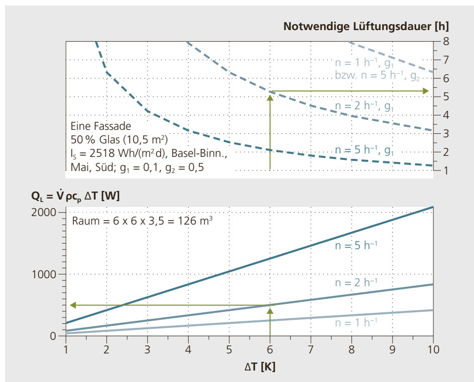
Abbildung 2.28: Kühlpotenzial durch Lüftung.
