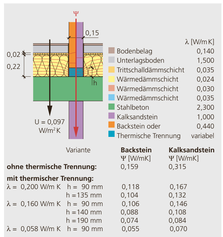
Abbildung 3.28: Wenn die Wand von der Stahlbetondecke thermisch getrennt werden kann, ist es optimal, die gesamte Wärmedämmschicht über der Decke anzuordnen. Je höher das thermisch trennende Element und je kleiner dessen Wärmeleitfähigkeit, desto kleiner wird der Wärmebrückenverlust bei diesem Bauteilübergang. In der Praxis bestimmen die statischen Kriterien über die Einsatzmöglichkeit solcher Elemente (z.B. Thermur, Ytong-Thermofuss, Foamglas-Perinsul).
