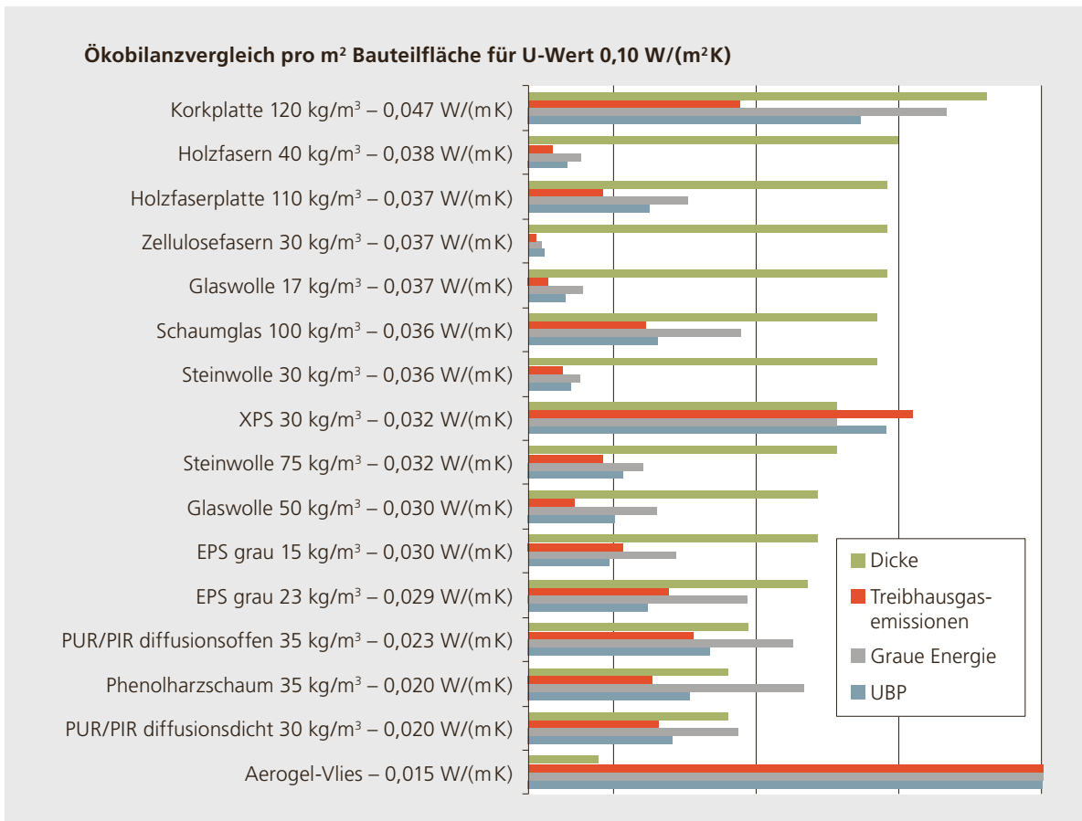
Abbildung 2.6: Umweltbelastung verschiedener Wärmedämmstoffe, referenziert auf einen U-Wert von 0,10 W/(m 2 K). Stand 10/2019. (Quellen: KBOB – Ökobilanzdaten im Baubereich und SIA-Baustoffkennwerte)
