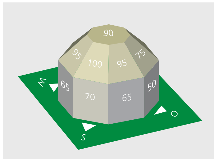
Abbildung 4.36: Abhängigkeit der Stromproduktion von PV-Modulen von der Orientierung und dem Neigungswinkel. (Quelle: Swissolar)
