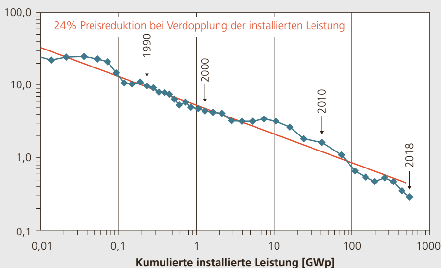
Mittlerer Preis PV-Module in Europa/Wp, 2018 [Euro pro Watt]
