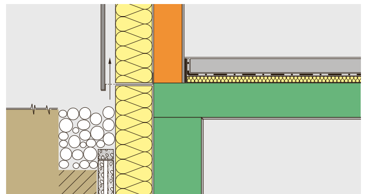
Abbildung 3.18: Perimeterdämmung im Erdreich als Fortsetzung einer Aussendämmung verputzt oder mit hinterlüfteter Bekleidung.
