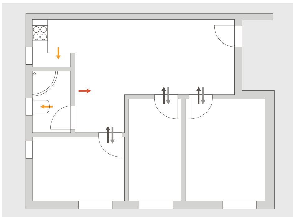
Abbildung 4.16: Prinzip der Verbundlüftung bei einer Wohnung.
