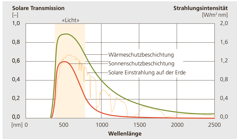
Abbildung 2.22: Selektivität. Beispiel der wellenlängen-abhängigen solaren Transmission einer Wärmeschutzbeschichtung (Interpane Iplus S) sowie einer Sonnenschutzbeschichtung (Interpane 52/29), jeweils auf einem 6-mm-Flachglas.
