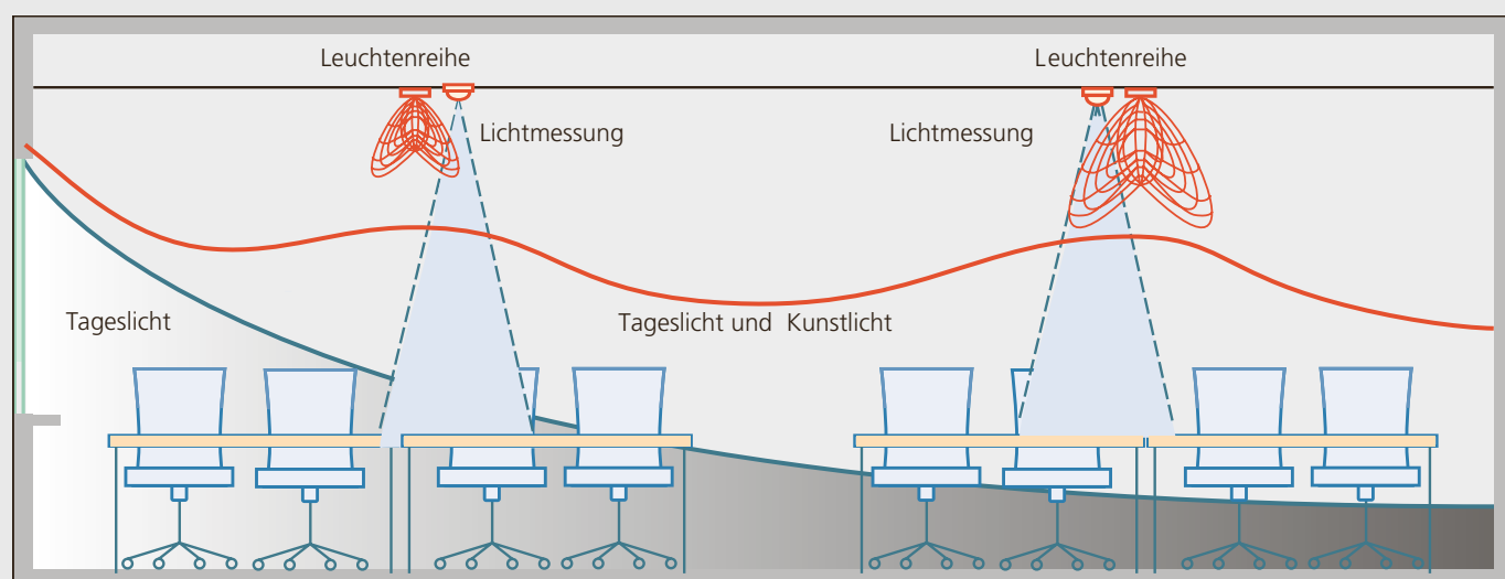
Abbildung 4.32: Verlauf der Beleuchtungsstärke des Tageslichts (blau) und der zugeschalteten elektrischen Beleuchtung (rot) eines einseitig befensterten Klassenraums. (Quelle: Trilux)
