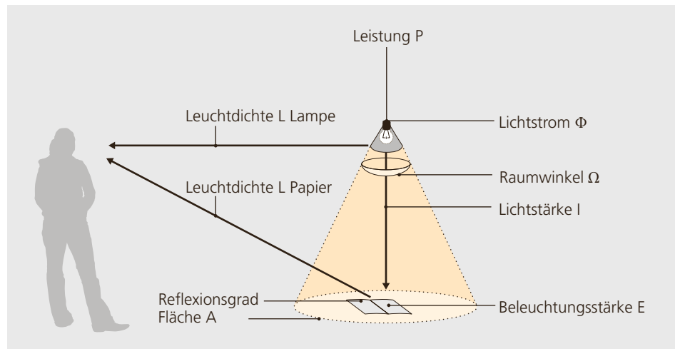
Abbildung 4.25: Zusammenhang der lichttechnischen Grössen. (Quelle: vdf Hochschulverlag)
