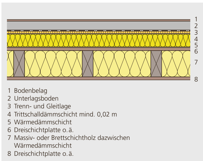
Abbildung 3.21: Bodenkonstruktion über Holzbalkendecke, mit Wärmedämmschicht zwischen den Holzbalken und variablen Wärme-/Trittschalldämmschichten über der Holzbalkendecke, je nach Anforderung an den Wärme- und Trittschallschutz.
