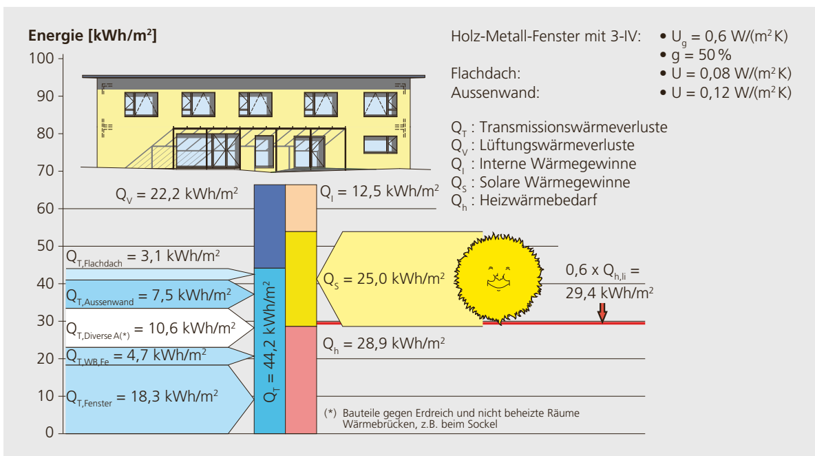
Abbildung 3.1: Energiebilanz einer hochgedämmten Gebäudehülle. Die Fenster verursachen, zusammen mit den Wärmebrücken beim Einbau, über 50% der Transmissionswärmeverluste. Der nutzbare Anteil der Energiegewinne durch Sonneneinstrahlung ist aber noch deutlich grösser als die gesamten Verluste beim Fenster. WB: Wärmebrücken
