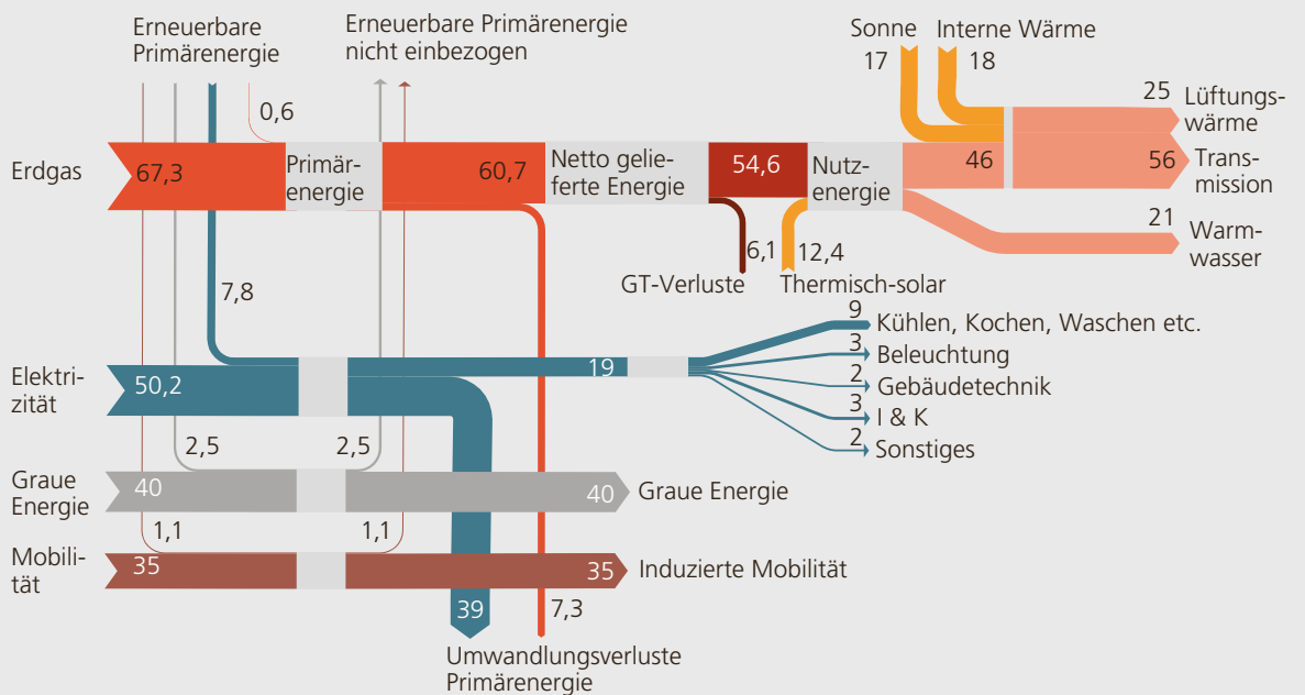
Abbildung 1.6: Spezifische Energieflüsse in kWh pro m 2 EBF pro Jahr in einem durchschnittlichen Mehrfamilienhaus-Neubau mit einem Erdgas-Wärmeerzeuger für Heizung und Warmwasser.
