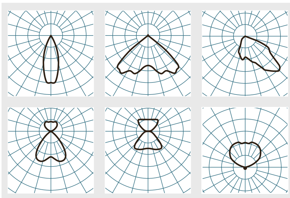
Abbildung 4.29 : Beispiele verschiedener Lichtstärkeverteilungskurven (oben von links nach rechts): tief strahlend, breit strahlend, asymmetrisch strahlend, unten von links nach rechts: vorwiegend direkt strahlend, gleichförmig strahlend, indirekt strahlend. (Quelle: Trilux)
