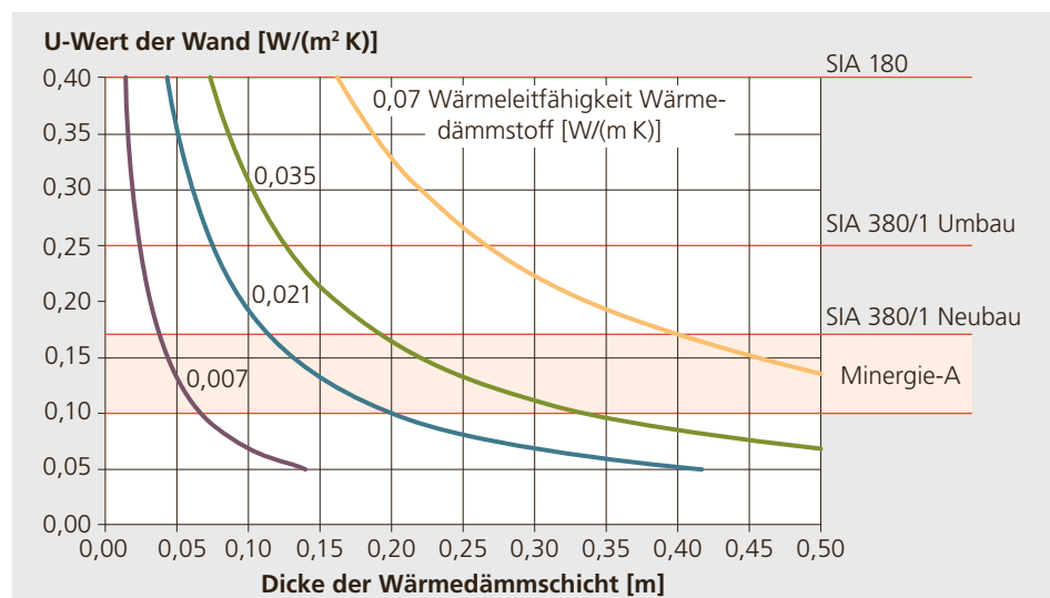
Abbildung 2.4: Erforderliche Wärmedämmdicken gegen Aussenklima in Abhängigkeit zur Wärmeleitfähigkeit des Wärmedämmstoffs.
