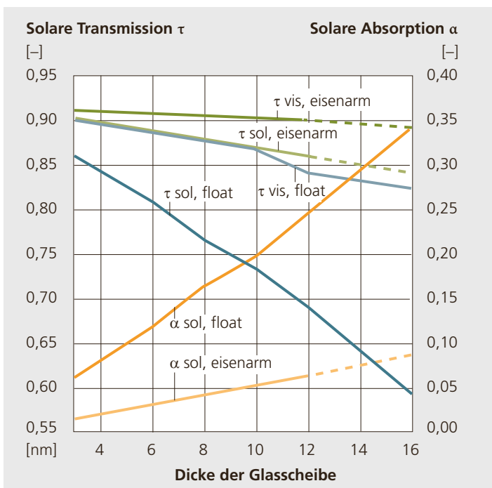
Abbildung 2.24: Solare Transmission und Absorption ( \tau_{sol} , \alpha_{sol} ) sowie Lichttransmission und Lichtabsorption ( \tau_{vis} , \alpha_{vis} ) in Abhängigkeit der Glasstärke. Gezeigt sind Werte für Flachglas («float») und eisenarmes Glas.
