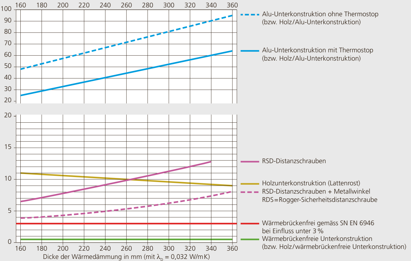
Abbildung 3.5: Beispiele für die in etwa zu erwartende prozentuale Erhöhung des U-Wertes durch verschiedene Unterkonstruktionssysteme, abhängig von der Unterkonstruktion und der Dicke der Wärmedämmung, bei Verankerungsgrund aus Stahlbeton. Differenzen von weniger als 3% zwischen dem U-Wert ohne und mit Wärmebrückeneinfluss, wie dies z. B. bei Wärmedämmkonsolen der Fall ist, müssen gemäss SN EN 6946 nicht berücksichtigt werden. Bei Distanzschrauben resultiert, je nach System und Dicke der Wärmedämmschicht, eine Erhöhung des Wärmeabflusses um etwa 3% bis 15%. Bei Holzunterkonstruktionen ist der Wärmebrückeneinfluss abhängig vom Holzanteil (6% berücksichtigt) und er nimmt infolge Überdämmung der Holzquerschnitte mit zunehmender Wärmedämmschichtdicke ab; er beträgt etwa 9% bis 11%. Bei Alu-Unterkonstruktionen beträgt der Wärmebrückeneinfluss mindestens 20% und er kann bis fast zu einer Verdoppelung des Wärmedurchgangs führen. Mit stockwerkübergreifenden Alu-Unterkonstruktionen können jedoch erheblich kleinere Wärmebrückenverluste erreicht werden als bei «normalen» Alu-Unterkonstruktionen. Grundsätzlich sind die effektiven Wärmebrückenverluste zur Ermittlung der korrekten Wärmeverluste (U-Werte) objektspezifisch zu beurteilen.
