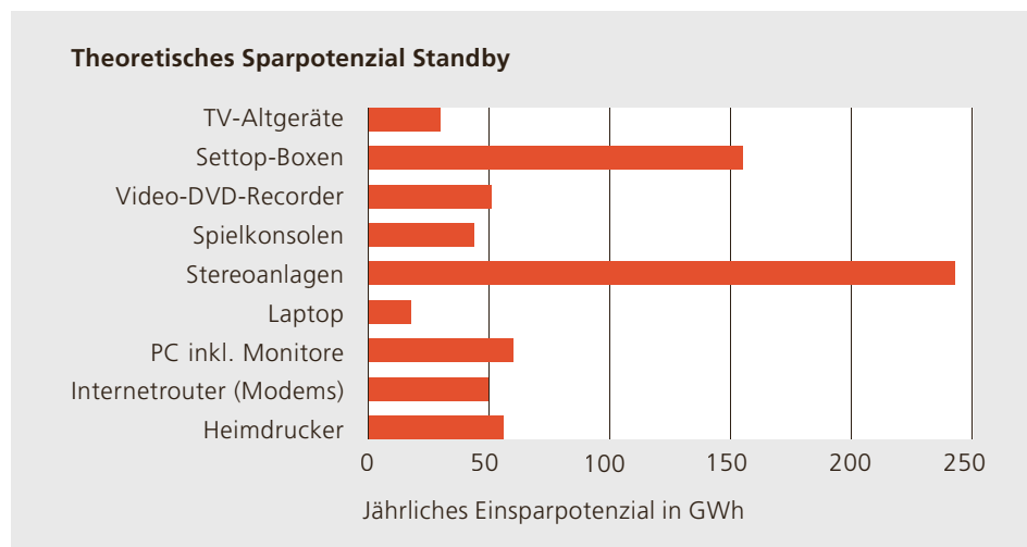
Abbildung 4.23: Theoretisches Einsparpotenzial Standby [13].
