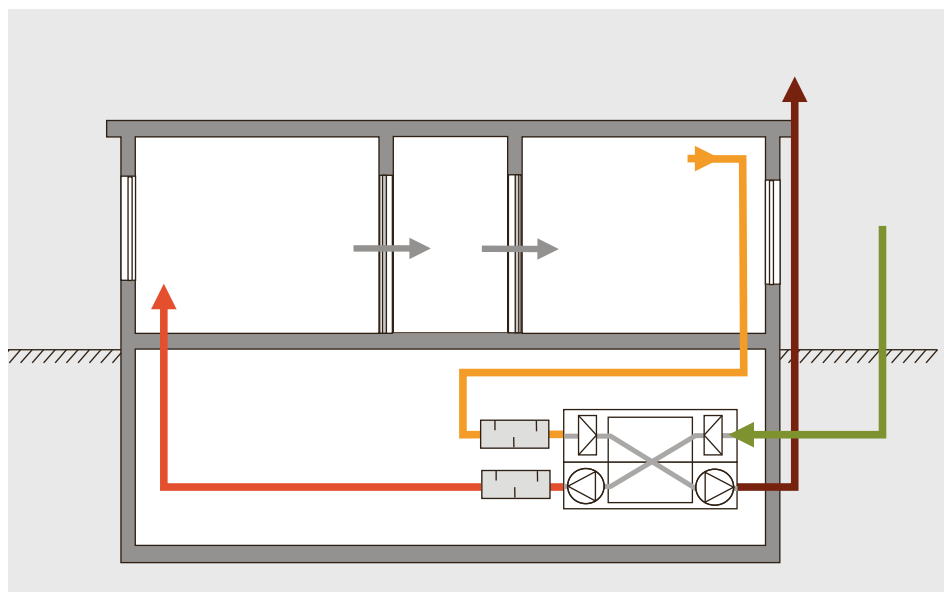
Abbildung 4.10: Prinzip Komfortlüftung.
