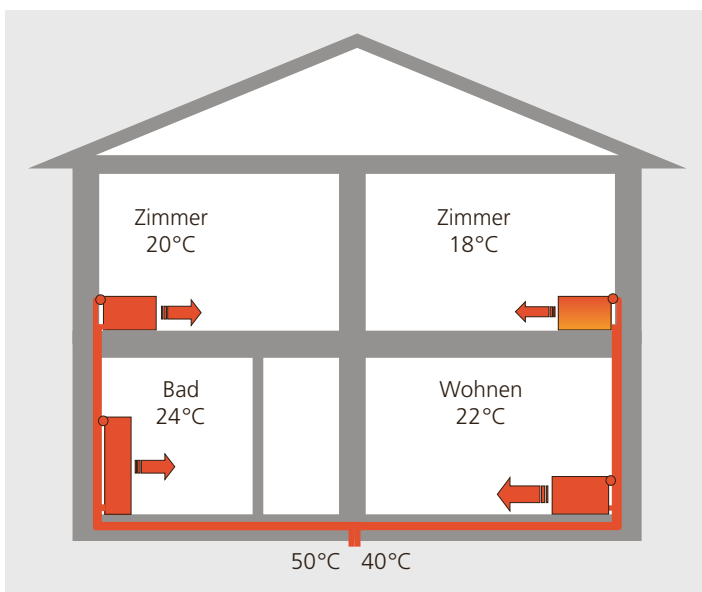
Abbildung 4.1: Prinzip Wasser- heizung mit Heiz- körpern.
