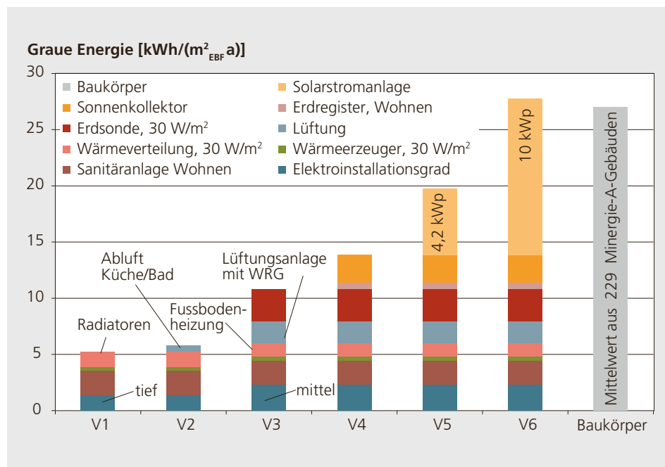
Abbildung 1.25: Graue Energie von verschiedenen Ausbaugraden der Gebäudetechnik im Vergleich zum Baukörper (Basis KBOB-Ökobilanzdatenbank 2012).
