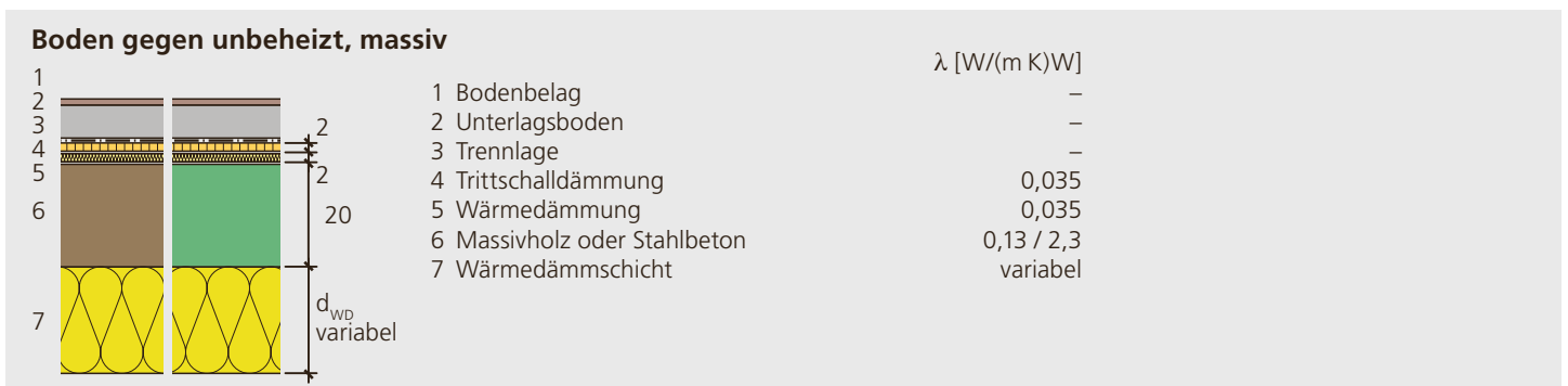
Abbildung 2.14: Boden gegen unbeheizt, massiv.
