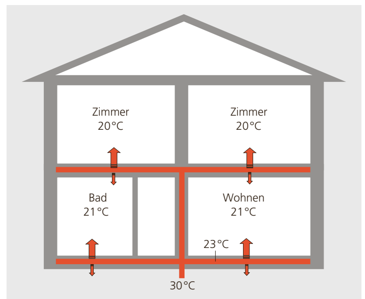
Abbildung 4.2: Prinzip Wasser- heizung mit Fuss- bodenheizung oder TABS.
