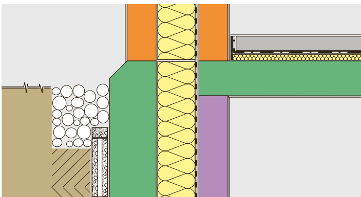
Abbildung 3.19: Zweischalenmauer- werk im Erdreich als Fortsetzung eines Zweischalen-Sicht- mauerwerks.
