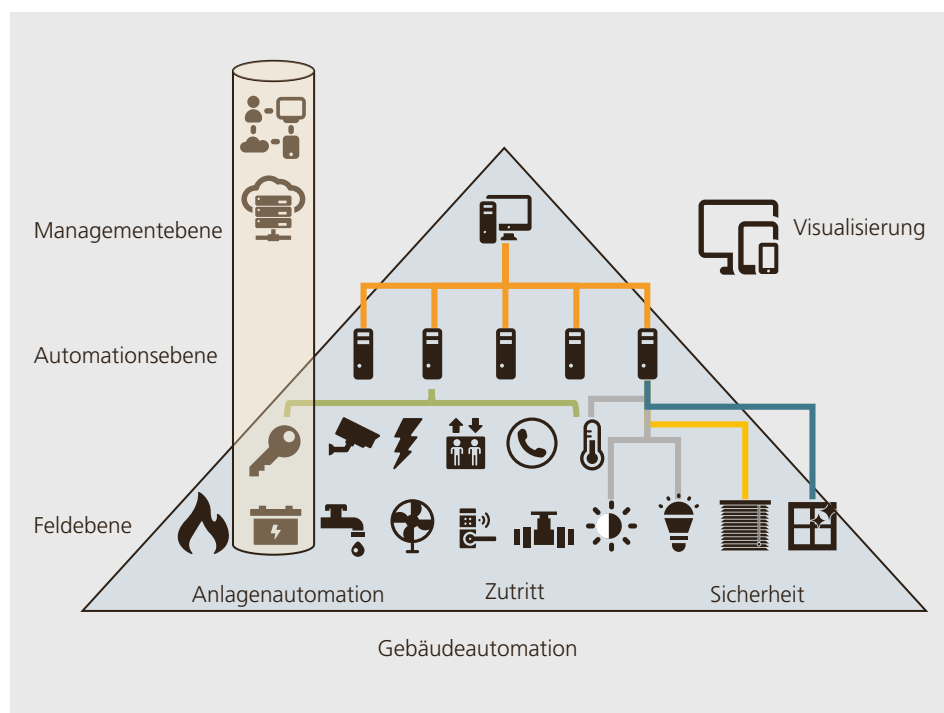
Abbildung 4.44: Nach EN 16484 wird die Gebäudeautomation in die Feld-, Automations- und Managementebene eingeteilt. Dies gilt jeweils einzeln, beispielsweise für die Sicherheit und die Heizungsanlage. In Wohnbauten interagieren die einzelnen Gewerke nicht miteinander. Dies führt unter dem Blickwinkel «Optimierung Energiebedarf» zu suboptimalen Lösungen. Heute wird die Visualisierung häufig in eine Cloud ausgelagert und die Daten sind hiermit weltweit verfügbar; dieser Teil ist gelb hinterlegt. (Grafik: D. Kunz, FHNW)
