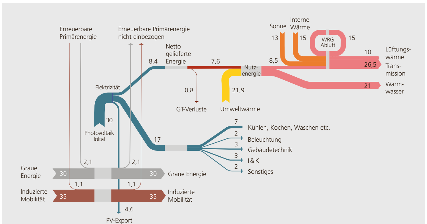
Abbildung 1.16: Spezifische Energieflüsse in kWh pro m 2 EBF und pro Jahr im Mehrfamilienhaus-Neubau, der die Standards Minergie-P und Minergie-A erreicht.
