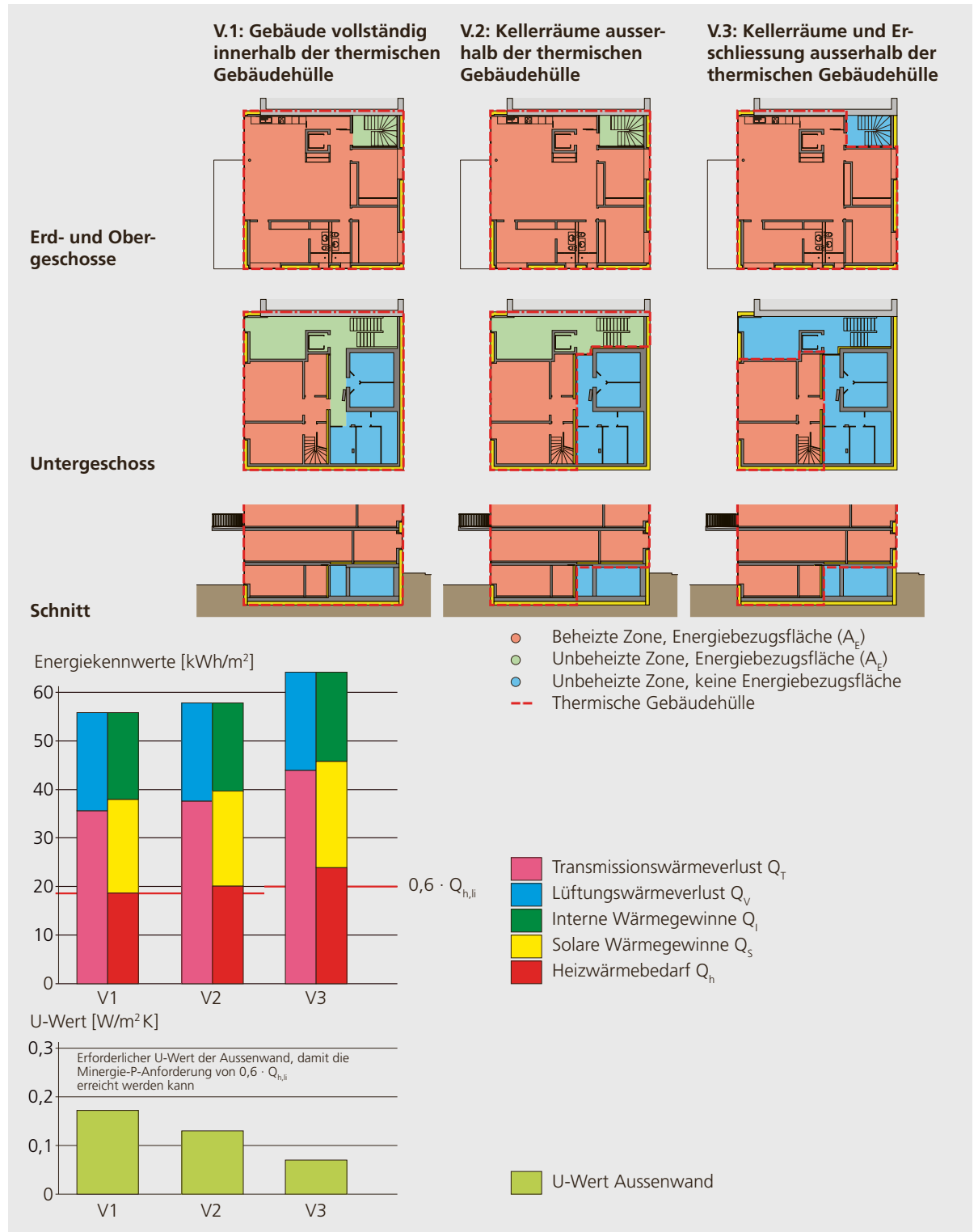
Abbildung 3.2: Die Wahl der thermischen Gebäudehülle beziehungsweise die Abgrenzung im und gegen das unbeheizte Untergeschoss ist wesentlich für den rechnerischen Nachweis des Heizwärmebedarfs. Eine thermische Gebäudehülle, die nur die aktiv beheizten Räume umfasst (vgl. V.3) hätte bei diesem Beispiel nie zum Ziel «Minergie-P» geführt, die Aussenwand hätte hierfür einen unrealistischen U-Wert von 0,07 \text{ W/(m}^2\text{K)} aufweisen müssen. Optimal zeigt sich bei diesem Objekt die Variante V.1, bei der sich sämtliche Räume innerhalb der thermischen Gebäudehülle befinden. Bereits mit einem U-Wert der Aussenwand von 0,172 \text{ W/(m}^2\text{K)} konnte der für Minergie-P erforderliche Heizwärmebedarf erreicht werden. Im Betrieb weisen natürlich alle drei Varianten denselben Heizwärmeverbrauch auf!
