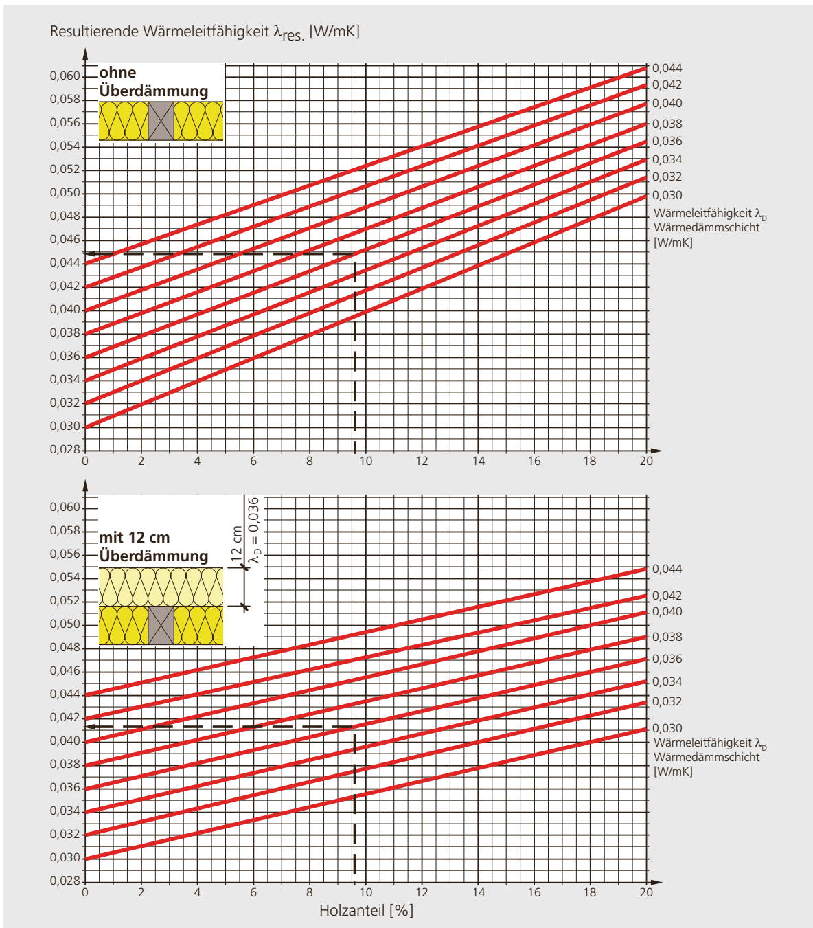
Abbildung 3.4: Resultierende Wärmeleitfähigkeit \lambda_{res.} für die inhomogene Schicht «Holz und Wärmedämmstoff» in Abhängigkeit vom Holzanteil und von der Wärmeleitfähigkeit \lambda_D des Wärmedämmstoffes, mit und ohne Überdämmung der inhomogenen Schicht. Bei 9,5% Holzanteil kann die resultierende Wärmeleitfähigkeit durch Überdämmung von \lambda_{res.} = 0,045 auf \lambda_{res.} = 0,041 W/mK reduziert werden.
