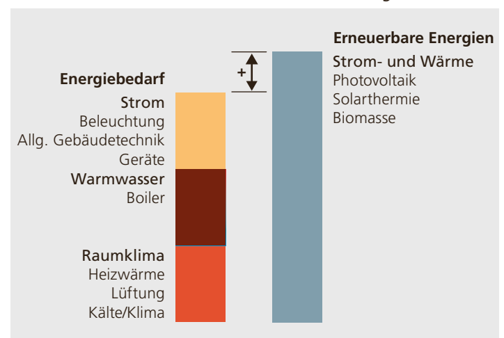
Abbildung 1.23: Schematische Darstellung der Plusenergiebilanz.
