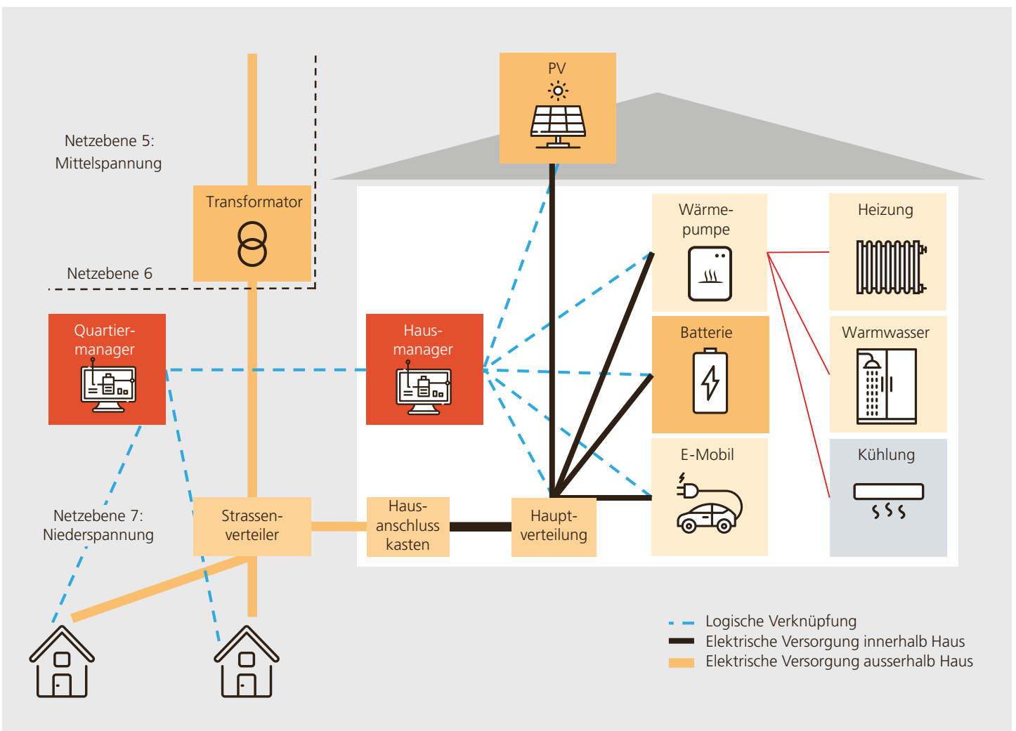
Abbildung 4.47: Die hierarchische Optimierung erfolgt dezentral in jedem Haus durch einen Hausmanager. Die übergeordneten Ziele des Quartiers werden in einem Quartiermanager optimiert und entsprechende Anreizsignale an die Hausmanager weitergegeben. (Quelle: D. Kunz, FHNW, Forschungsprojekt Energy Chance)
