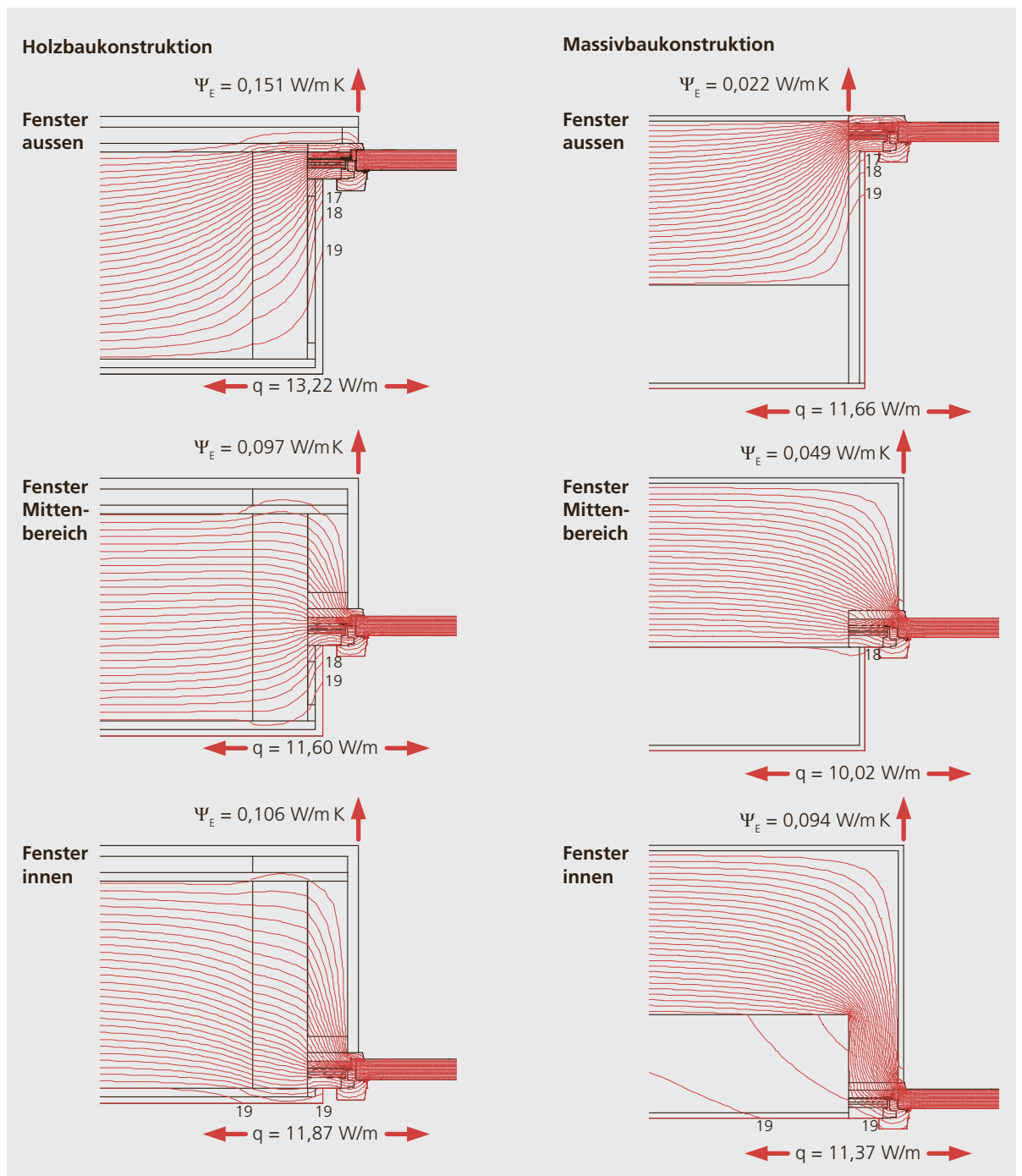
Abbildung 3.32: Wärmebrückenverlust \Psi_E beim seitlichen Fensteranschlag und Wärmeverlust q über den gesamten Detailperimeter (Wand mit U = 0,1 \text{ W/m}^2 \text{ K} ; Fensterrahmen mit U_f = 0,91 \text{ W/m}^2 \text{ K} ; Glas mit U_g = 0,5 \text{ W/m}^2 \text{ K} und \Psi_g = 0,05 \text{ W/m K} ). Der Fenstereinbau im Mittenbereich führt zu den kleinsten Energieverlusten. Der Fenstereinbau ganz innen zu maximal hohen inneren Oberflächentemperaturen. Beim ganz aussen angeschlagenen Fenster sind die Energieverluste am grössten, wobei sich dies wegen der veränderten Bezugsebenen nicht zwangsläufig im \Psi_E -Wert manifestiert.
