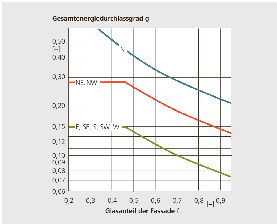
Abbildung 2.29: Anforderungen an den g-Wert von Fassadenfenstern (Verglasung und Sonnenschutz) je nach Glasanteil und Orientierung der Fassade. (Quelle: Norm SIA 180)
