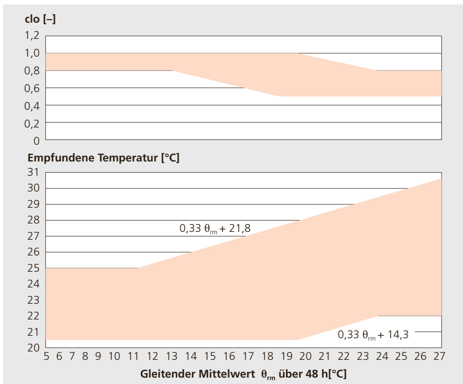
Abbildung 1.33: Anpassung der Kleidung (oben) und zulässige empfundene Temperatur für Räume mit natürlicher Belüftung, die weder geheizt noch gekühlt sind. Die empfundene Temperatur wird näherungsweise als arithmetisches Mittel der Raumlufttemperatur und der mittleren Strahlungstemperatur bestimmt. Der «clo»-Wert beschreibt die Wärmedämmwirkung der Bekleidung. (Quelle: nach SIA 180:2014)
