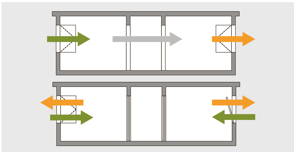
Abbildung 4.8: Querlüftung und einseitige Fenster- lüftung.
