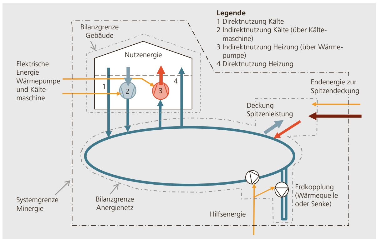
Abbildung 1.9: Anergienetz. (Quelle: Anwendungshilfe Minergie, www.minergie.ch)
