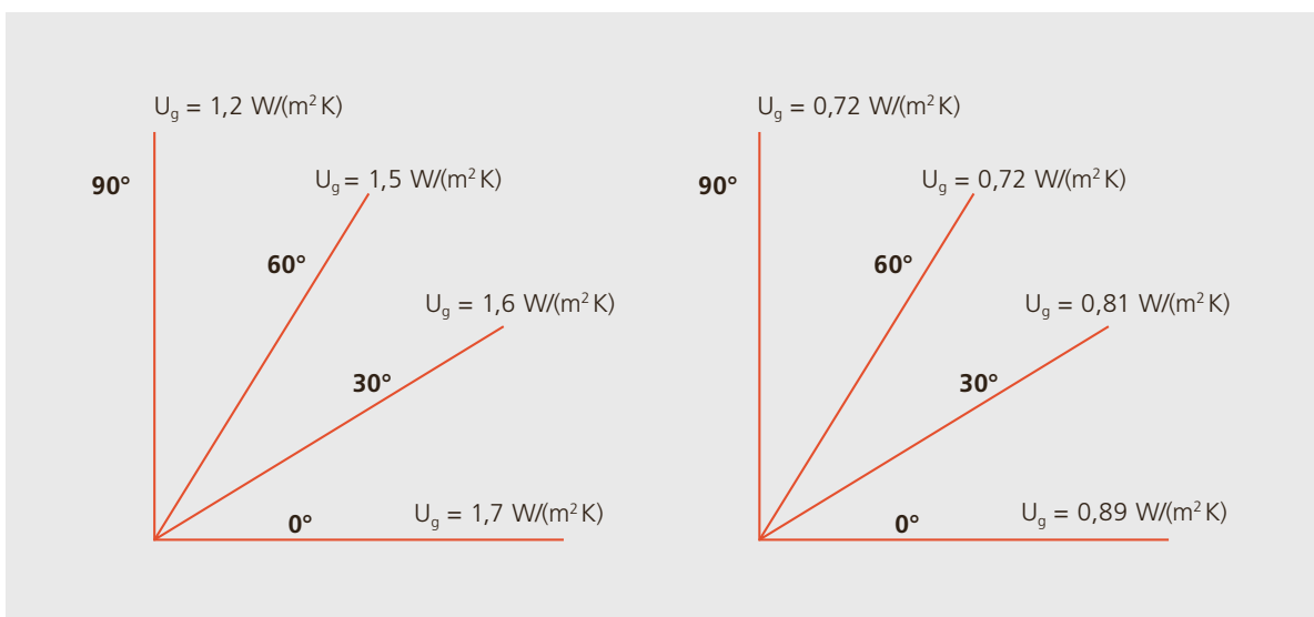
Abbildung 2.20: U_g -Wert in Abhängigkeit vom Neigungswinkel, links für eine Zweifach-, rechts für eine Dreifach-Isolierverglasung. (Quelle: ift Rosenheim)
