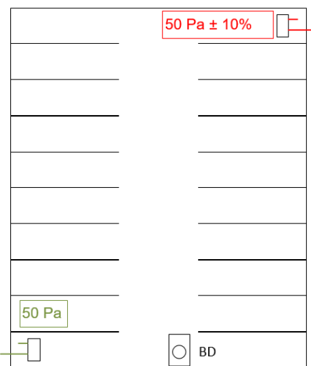
Abbildung 25: Grafik Überprüfung der Druckdifferenz zwischen innen und aussen in den kritischen Zonen; Beispiel Gebäudedruckdifferenz von 50 Pa am Einbauort der Messeinrichtung
