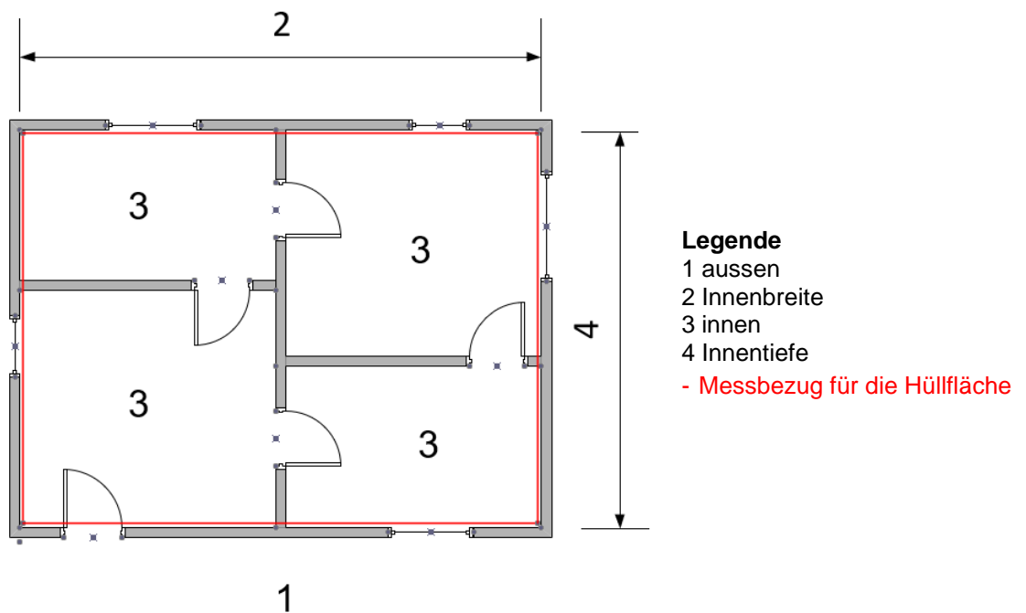
Abbildung 18: Grundriss mit Darstellung der Gesamt-Innenabmessungen (Quelle: SN EN ISO 9972; 2015)
