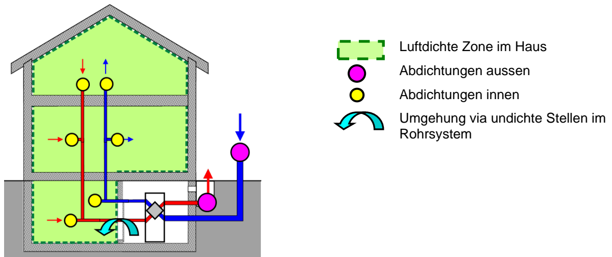
Abbildung 23: Mögliche provisorische Abdichtungen bei Lüftungsanlagen. (Quelle: Ingenieurbüro Baueck-Tanner)
