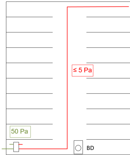
Abbildung 26: Grafik Überprüfung der Druckdifferenz innerhalb des Gebäudes; Beispiel Gebäudedruckdifferenz von 50 Pa am Einbauort der Messeinrichtung
