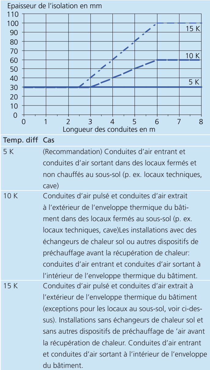
Epaisseur d'isolation minimale de conduites d'air, tuyaux et canalisations en présence d'une isolation thermique présentant une conductivité thermique de 0,03 W/mK < λ ≤ 0,05 W/mK [7]
