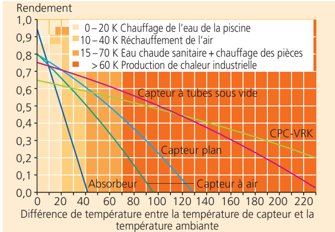
Chauffage solaire.
