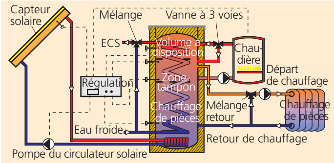
Chauffage solaire.
