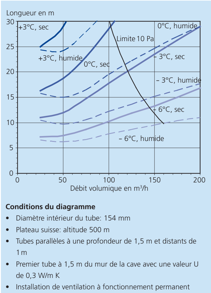
Plage d'utilisation de tubes de registres d'air géothermique avec un diamètre intérieur de 150 mm, conditions générales suivant l'encadré.
