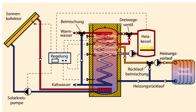
Solares Heizsystem
