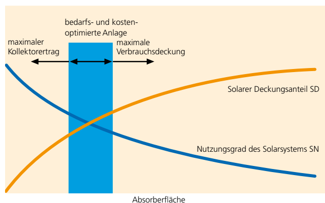
Sonnenkollektoranlagen können bezüglich Nutzungsgrad, Deckungsanteil oder Kosten optimiert werden.
