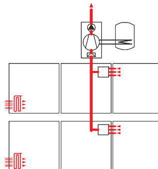
Installation d'extraction d'air avec PAC
