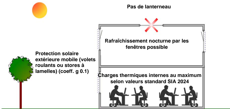
Figure 3 : Conditions cadres pour la variante 1
