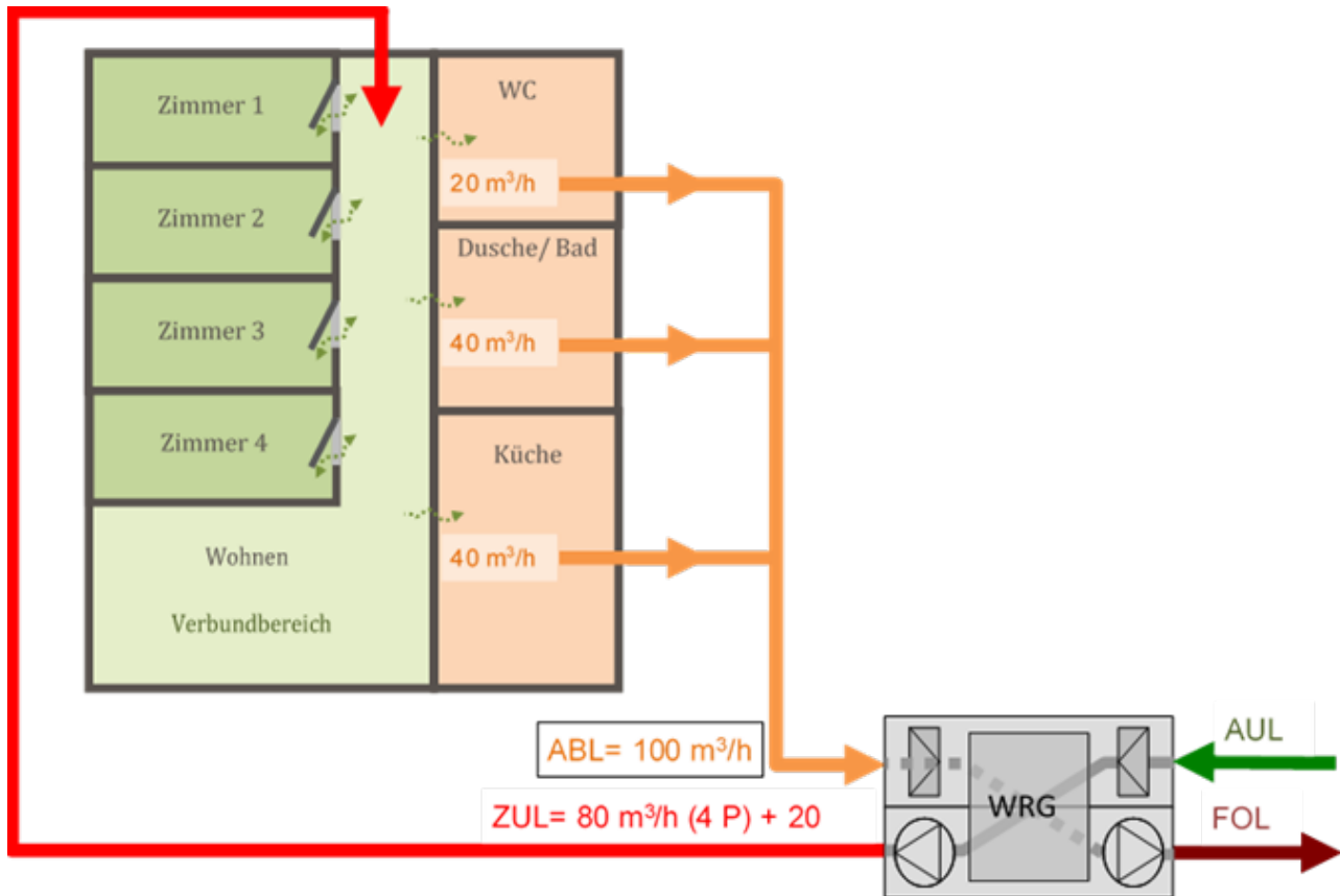
Abbildung 32: Beispiel Grundlüftung für Erneuerungen
