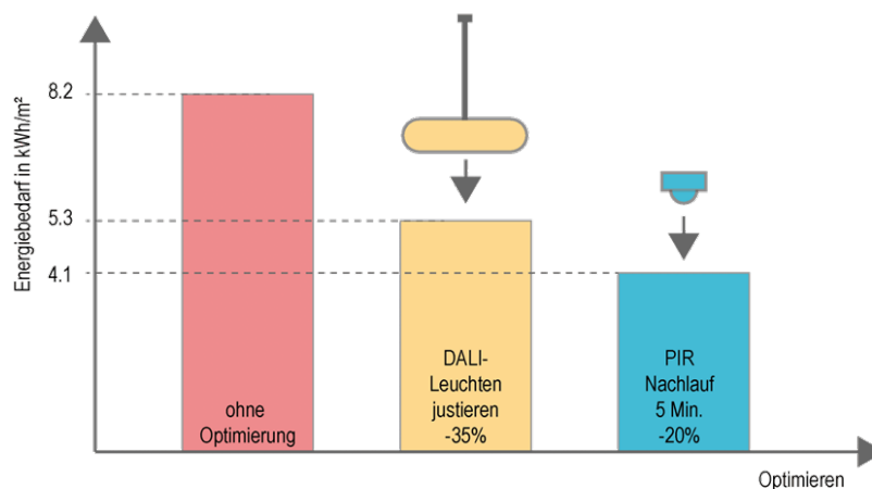
Abbildung 35: Beispiel «Optimierung Beleuchtung in einem Schulhaus»
