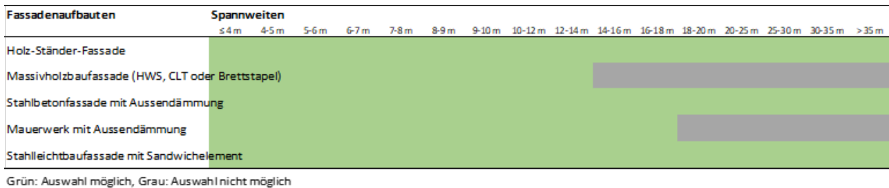
Abbildung 49: zeigt die möglichen Kombinationen zwischen Fassadenkonstruktionen und Spannweiten des Gebäudes. Grün = Auswahl möglich, Grau = Auswahl nicht möglich.
