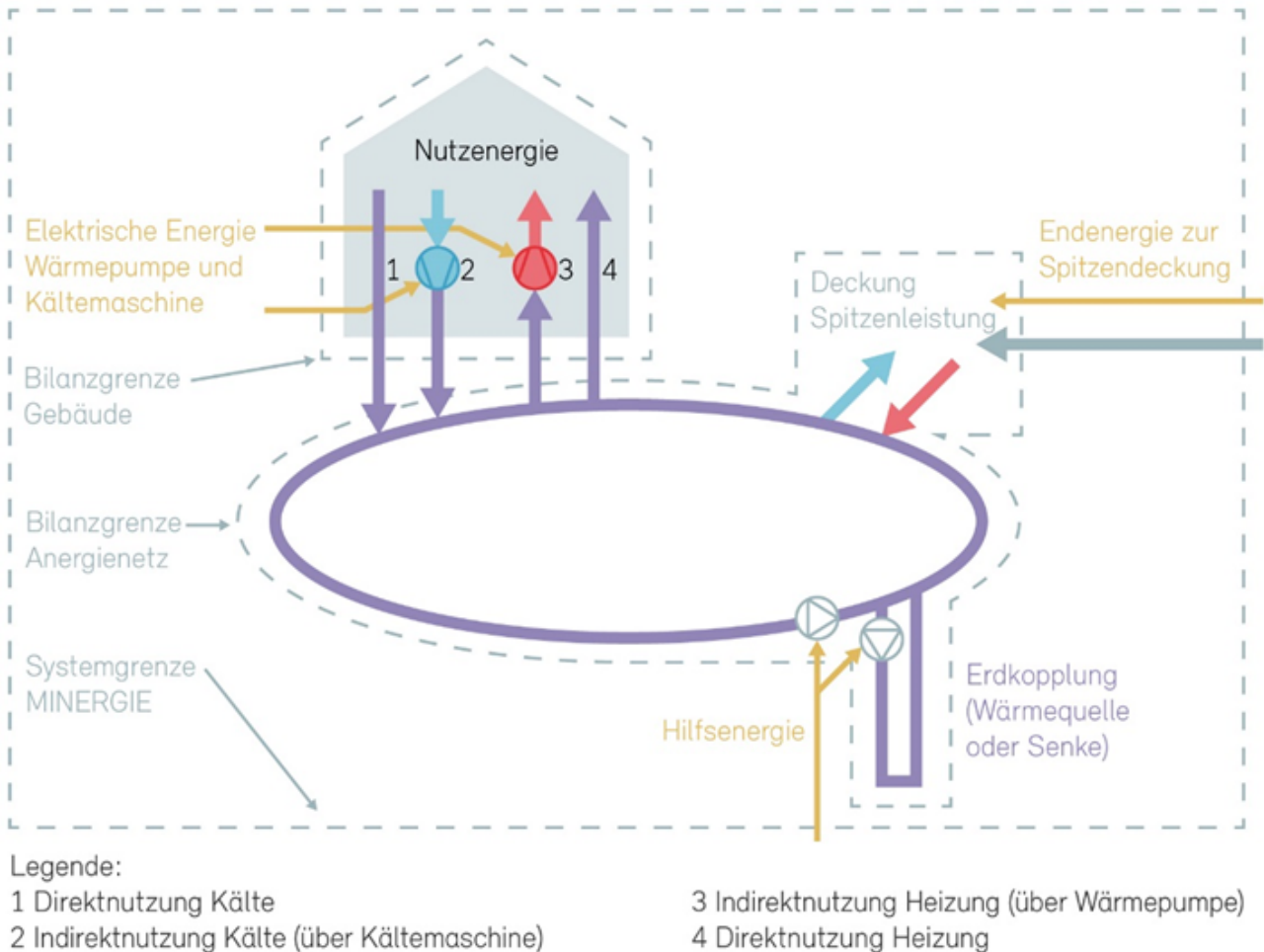
Abbildung 25: Prinzipskizze Anergienetz
