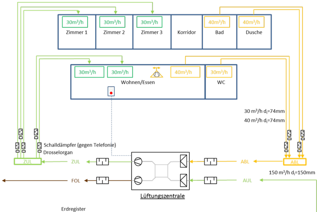
Abbildung 31: Beispiel Lüftungsschema für Kleinanlagen
