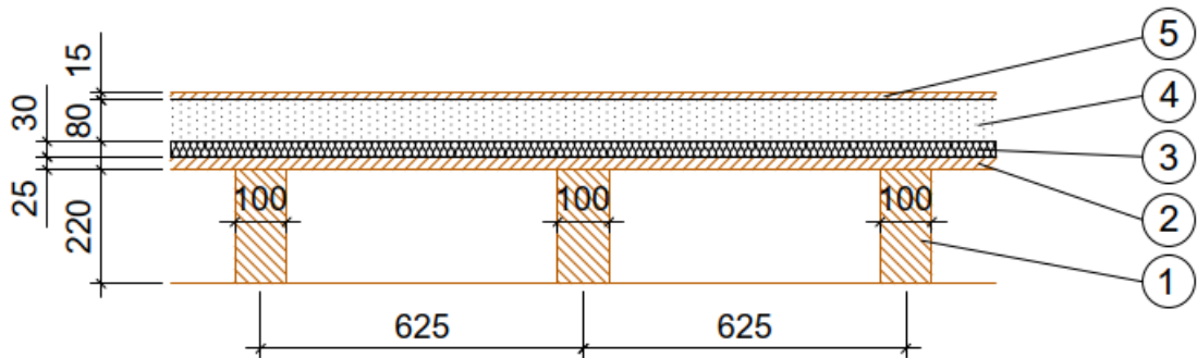
Abbildung 24: Aufbau Holzbalkendecke
