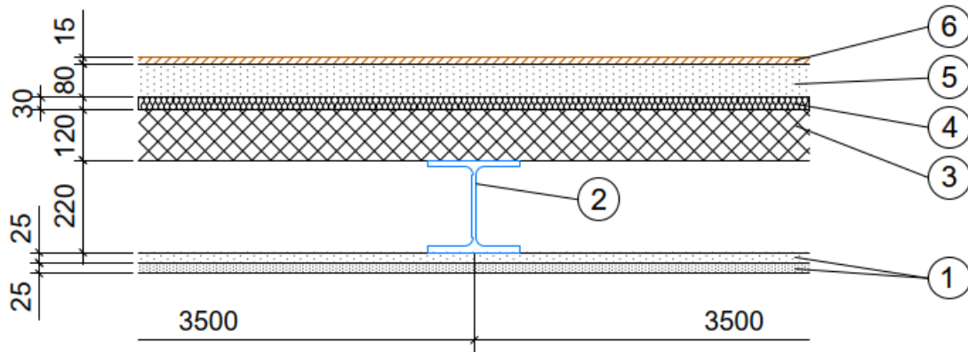
Abbildung 21: Aufbau Stahl-Beton-Verbunddecke
