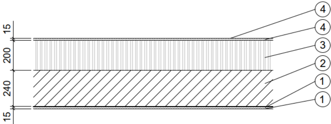
Abbildung 43: Mauerwerkfassade mit Kompaktfassade/Wärmedämmverbundsystem (WDVS)
