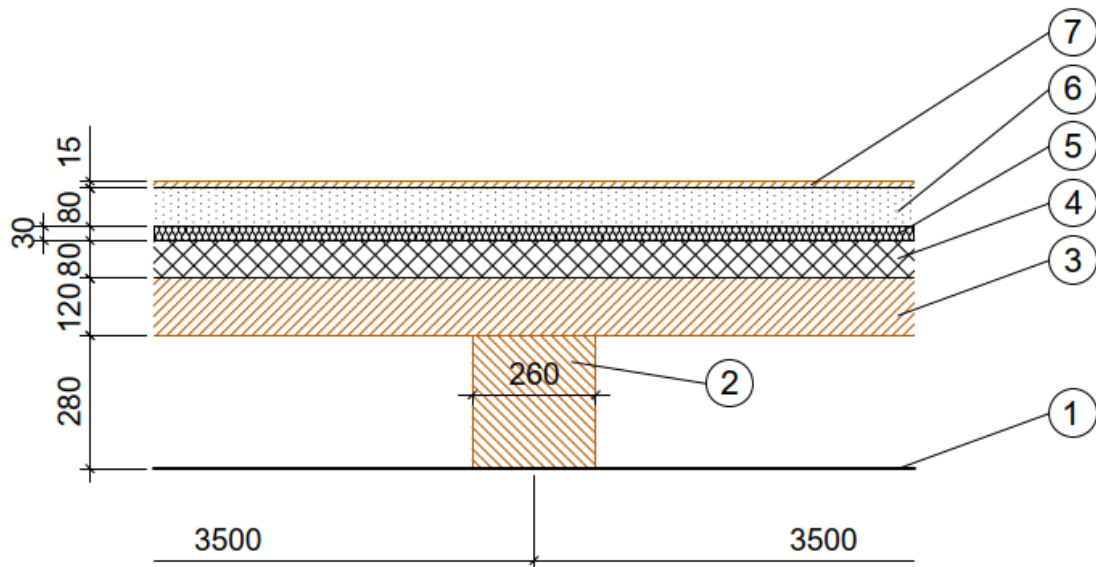
Abbildung 23: Aufbau Holz-Beton-Verbunddecke (Brettstapel)
