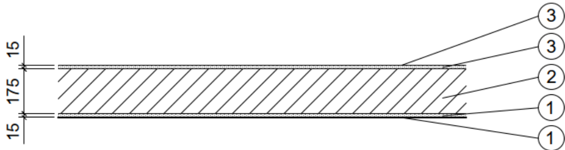
Abbildung 52: Aufbau Mauerwerkwand
