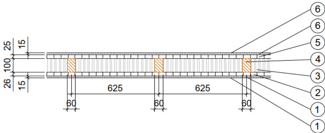
Abbildung 50: Aufbau Holz-Ständer-Wand
