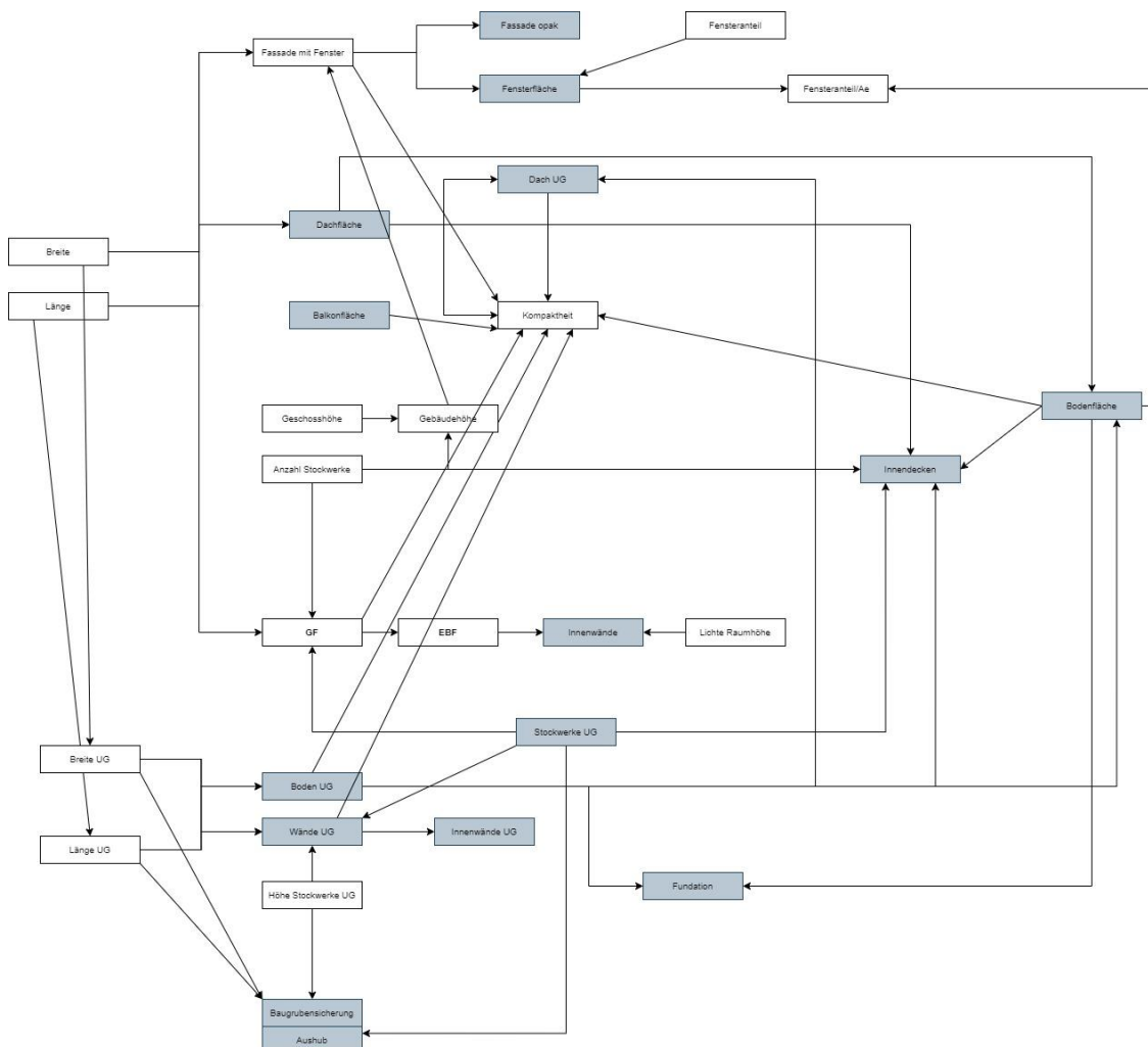
Abbildung 3: Abhängigkeiten zwischen den Bauteilflächen und den Gebäudedimensionen
