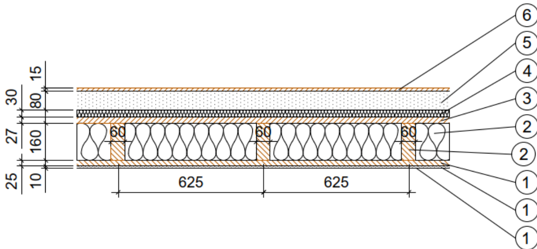
Abbildung 27: Aufbau Hohlkastendecke
