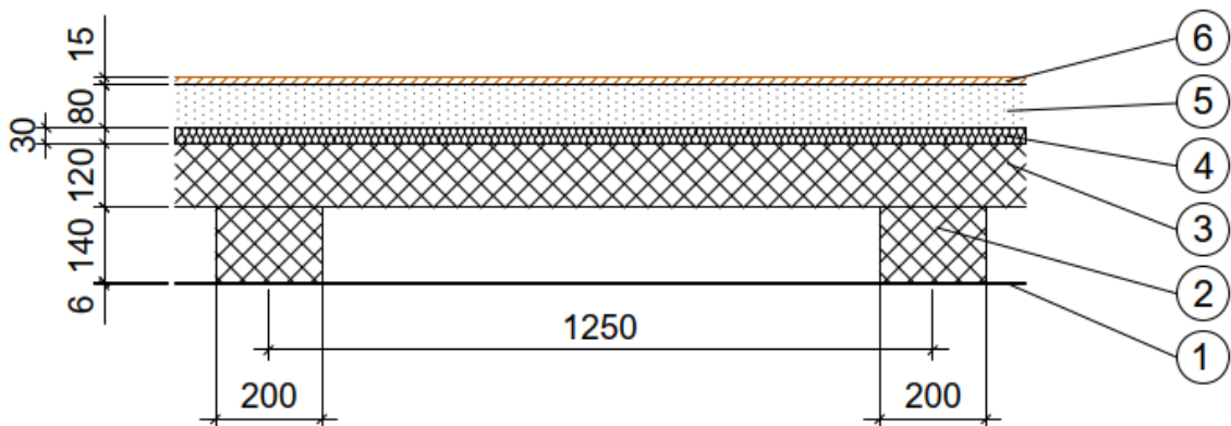
Abbildung 20: Aufbau Betonrippendecke
