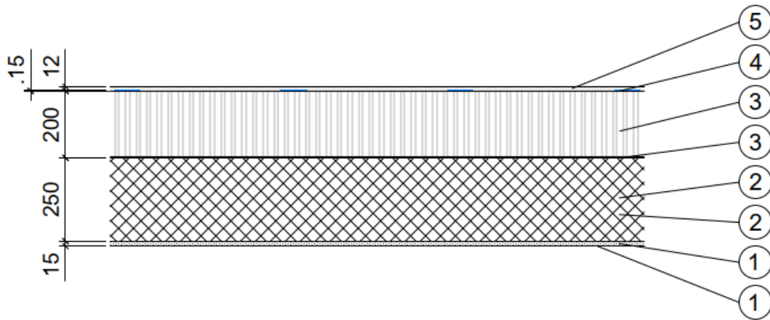
Abbildung 39: Stahlbetonfassade mit Aussendämmung, hinterlüftet mit Fassadenverkleidung aus Faserzement
