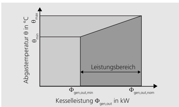
Abgastemperaturdiagramm
