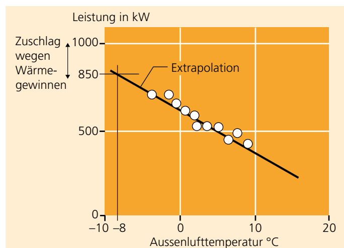
Leistungskennlinie aus einer Messung (Beispiel)
