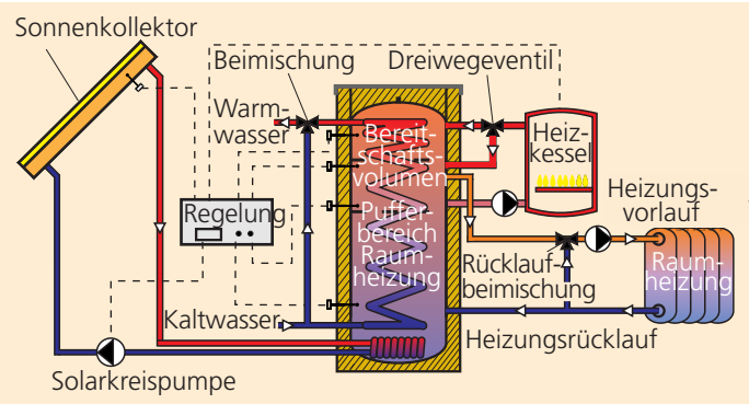
Solares Heizsystem
