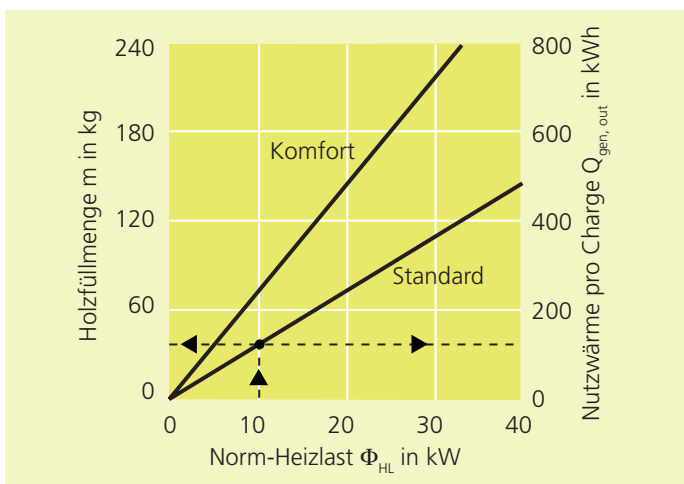
Auslegung Stückholzkessel
