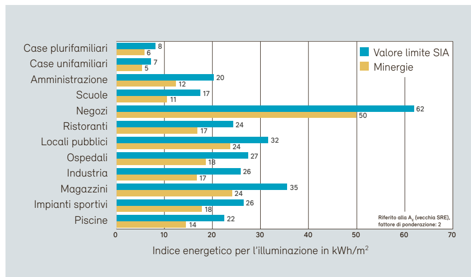
Parametri standard Minergie e valori limite SIA
