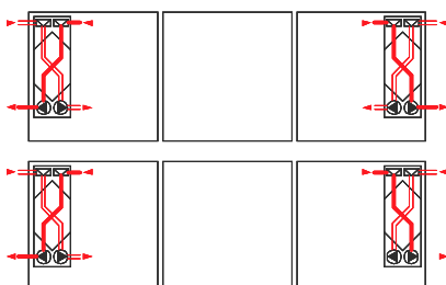
Installation d'extraction d'air avec prises d'air neuf
